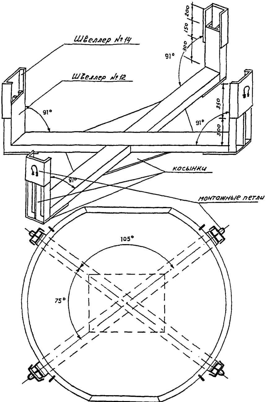
Рис. 4.1. Инвентарная оснастка для складирования и транспортировки оголовков
