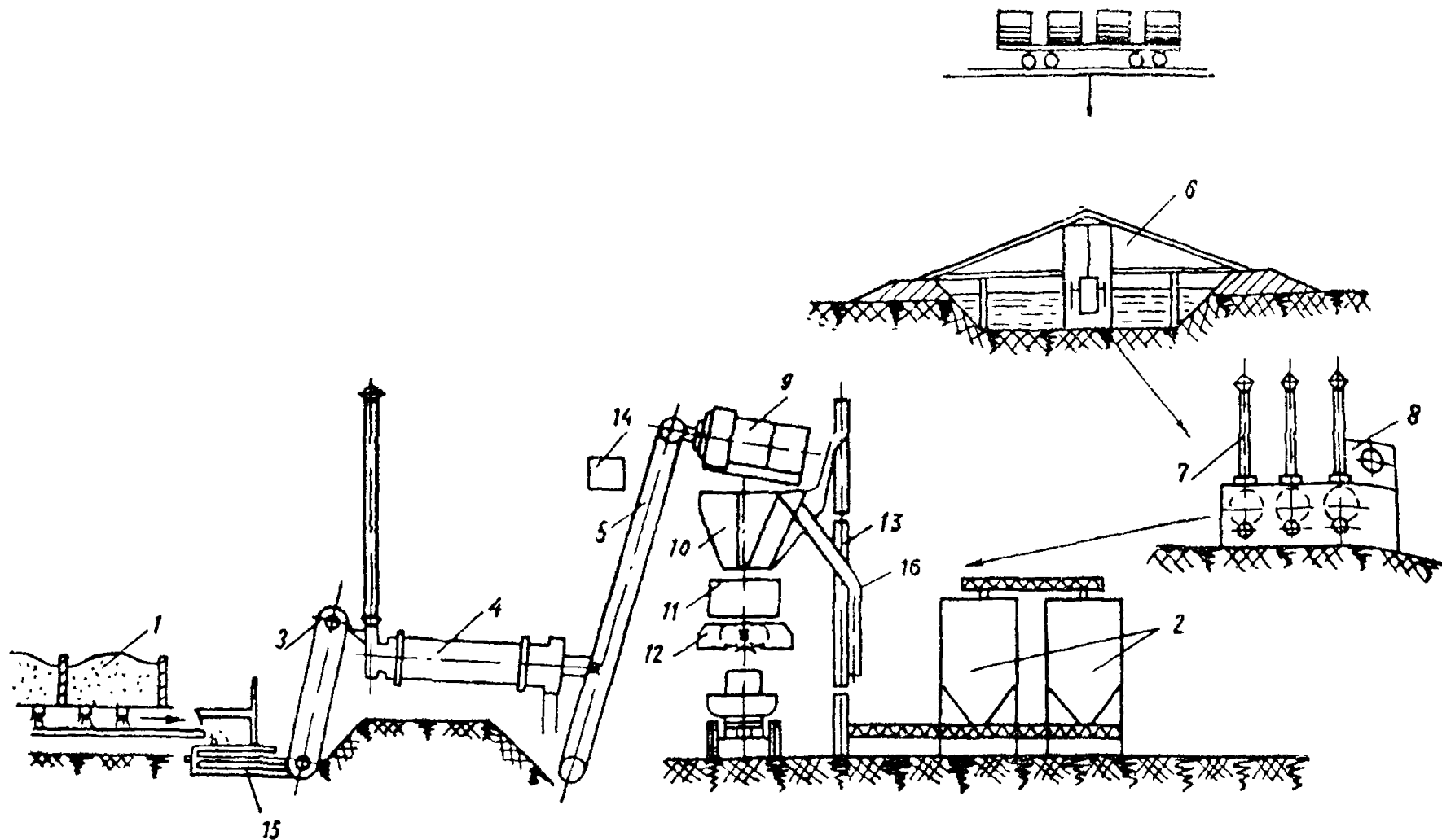
Технологическая схема АБЗ со смесителями Д-325 (Д-152):
