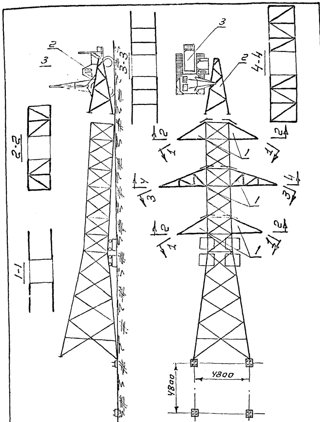
Рис. 7 Пристыковка траверсы и тросостойки к стволу опоры У110-2
