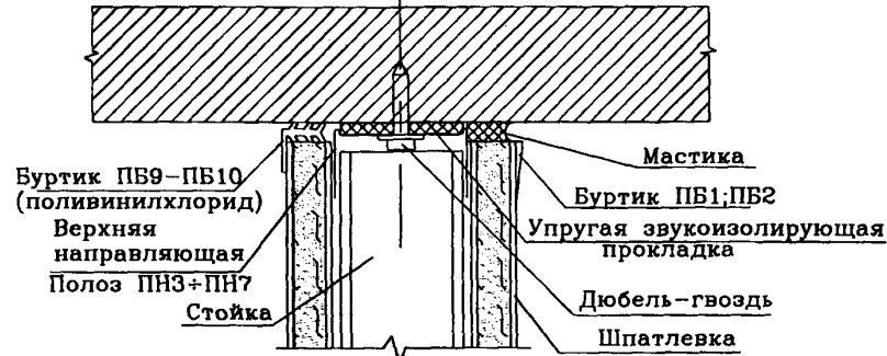
А) Узел примыкания перегородки к плите перекрытия.
