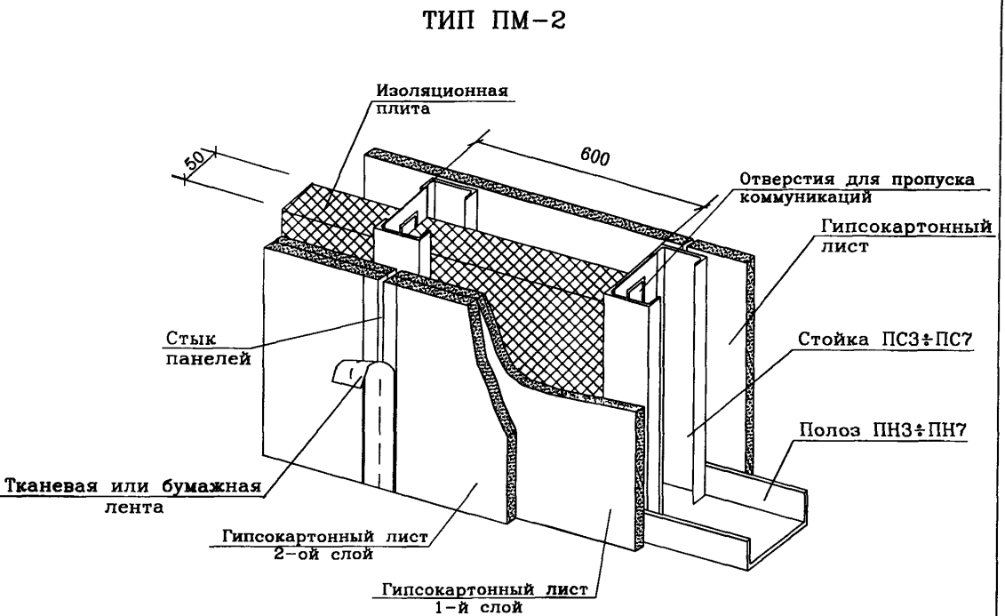
Рисунок 1 – Перегородки из гипсокартонных листов по металлическому каркасу.
