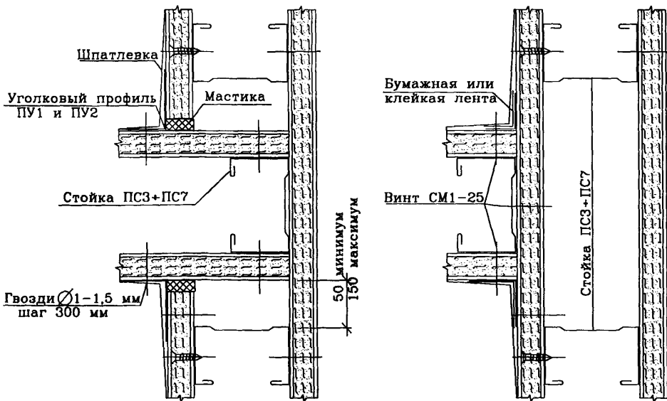
Рисунок 6 – Узлы примыкания перегородок.
