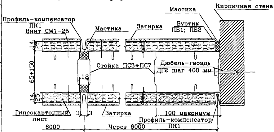
Е) Пересечение перегородок под прямым углом.
