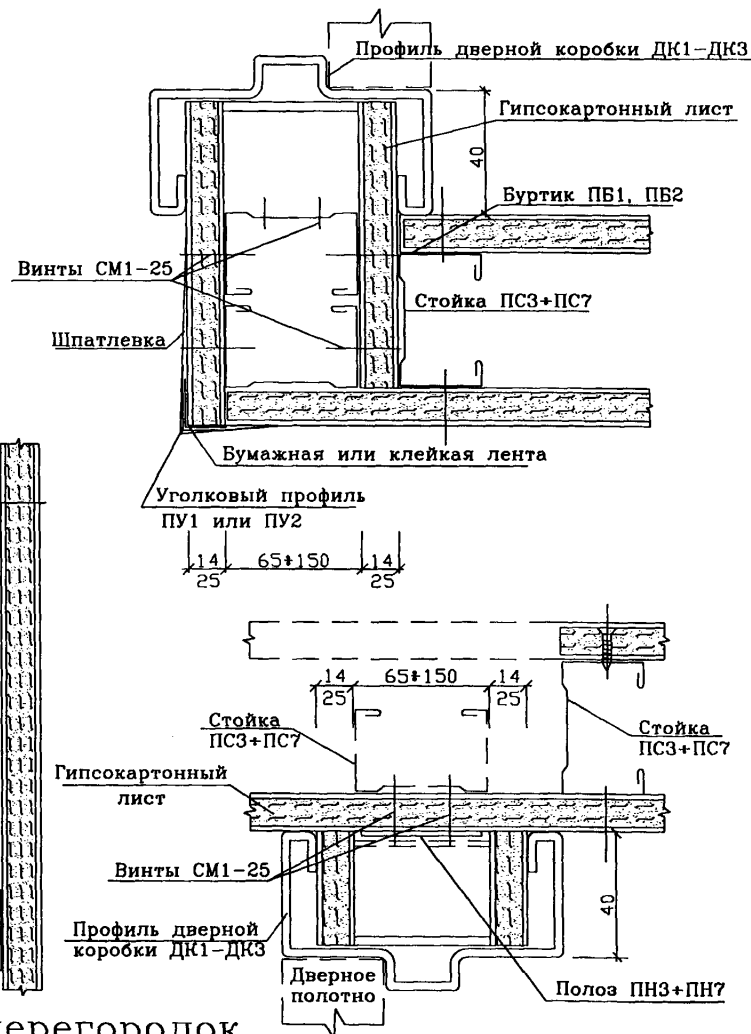
Ж) Варианты расположения дверных коробок в перегородках.
