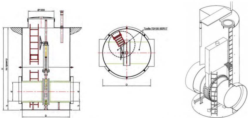
Рис.29. Колодец с шиберным затвором
