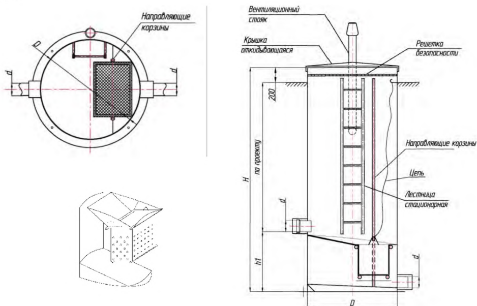
Рис.25. Конструкция колодца
