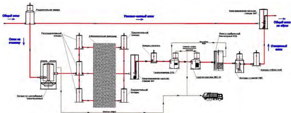
Схема №2.4 – технологическая схема оборудования
