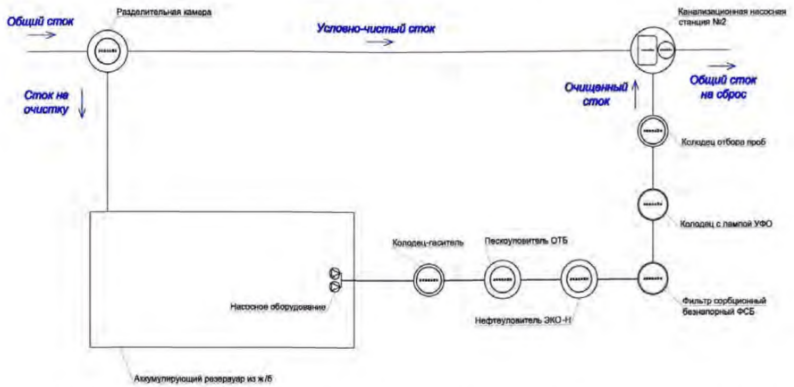
Схема №2.2 – применяется при больших объемах суточного стока, аккумуляционный резервуар выполняется из железобетона
