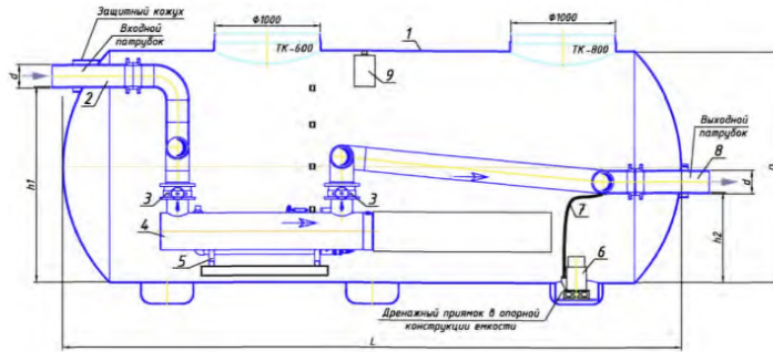
Рис.21. Горизонтальная конфигурация. Общий вид
