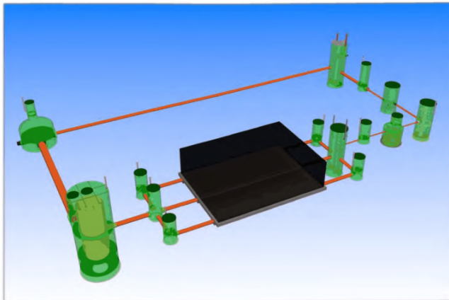
Схема №2.2 – применяется при больших объемах суточного стока, аккумуляционный резервуар выполняется из железобетона
