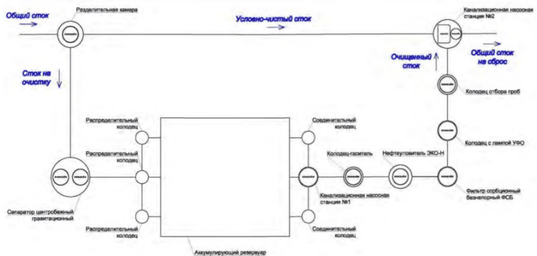
Схема №2.3 – применяется при больших объемах суточного стока, аккумуляционный резервуар выполняется по безбетонной технологии
