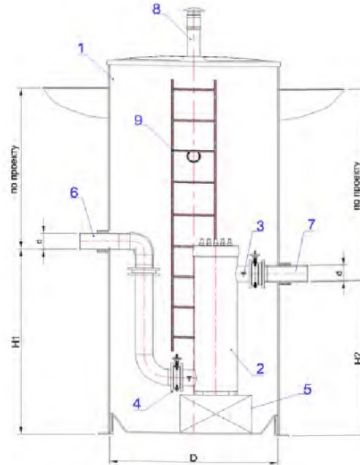
Рис.20. Колодец УФО (1-50 л/с)
