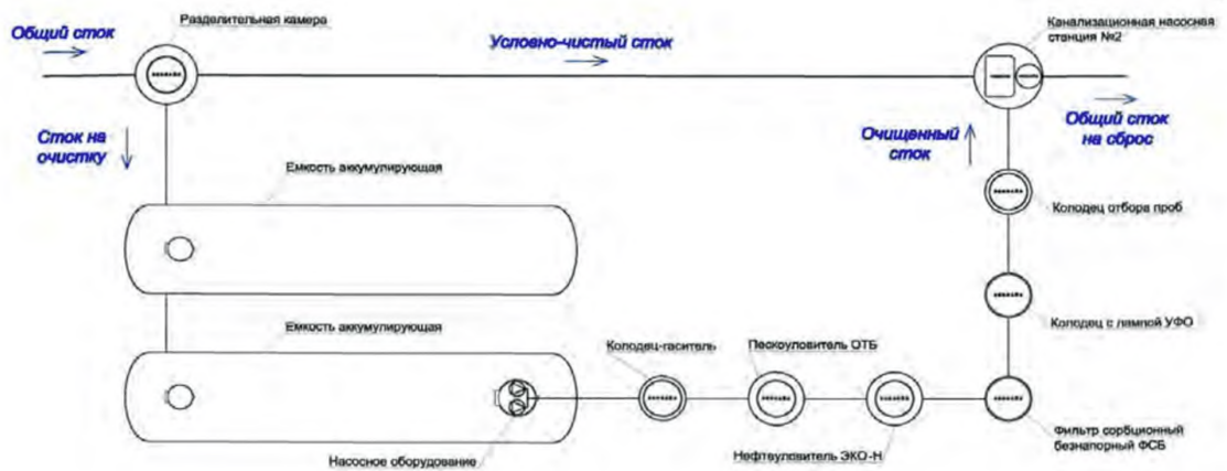
Схема №2.1 – применяется при небольших объемах суточного стока
