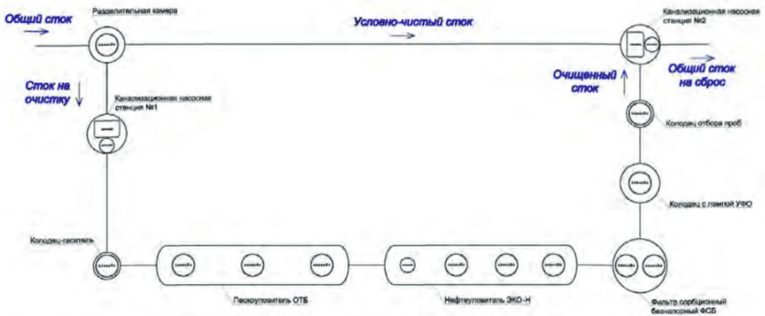
Схема №1.1 – применяется на расход очищаемого стока до 100 л/с
