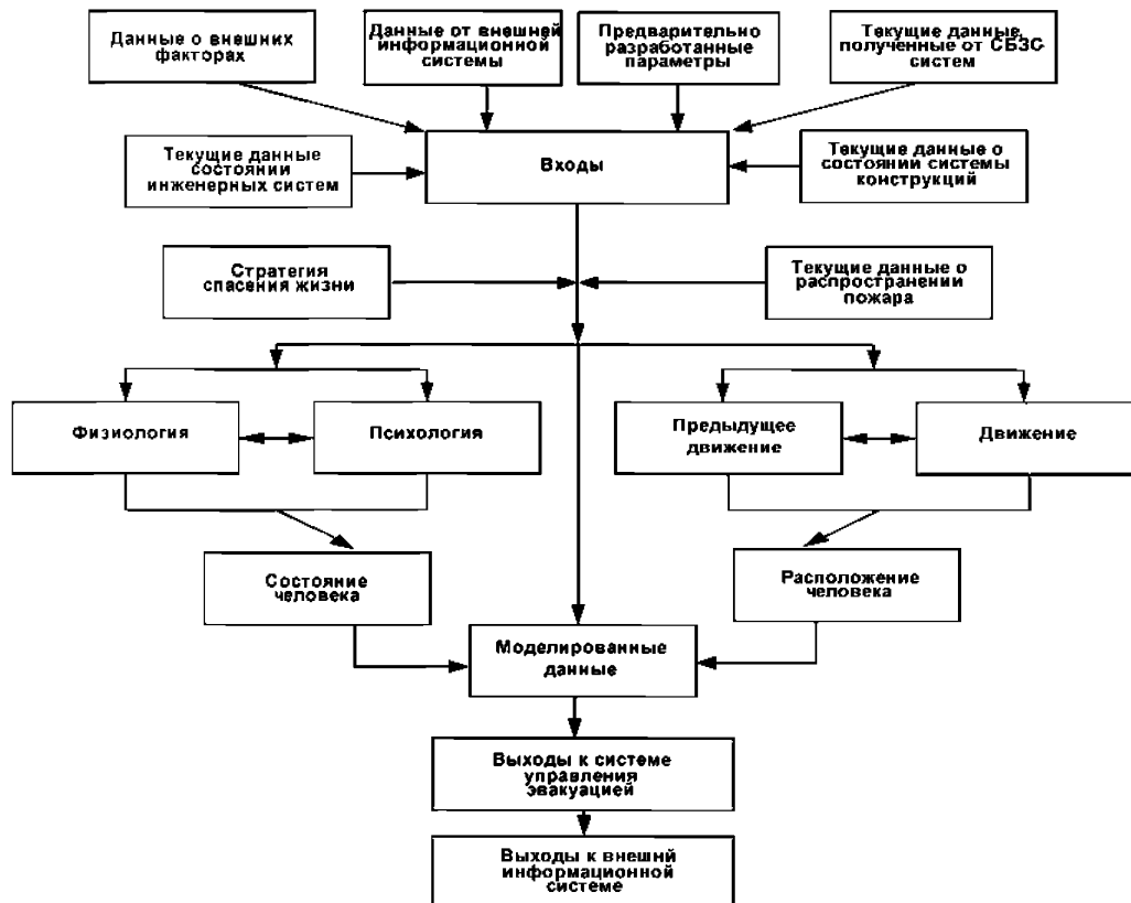
Рисунок Ж.1 – Динамическая модель управления эвакуацией людей при пожаре
