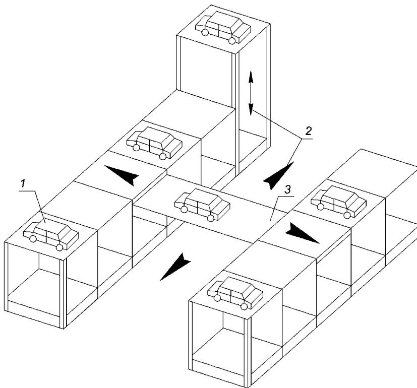
Рисунок А.5 – МПС многоуровневого типа
