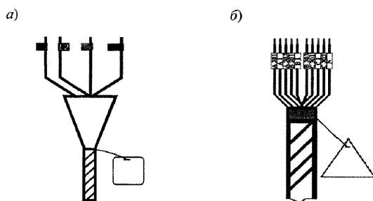
а) – силовые кабели до 1000 В; б) – контрольные кабели
