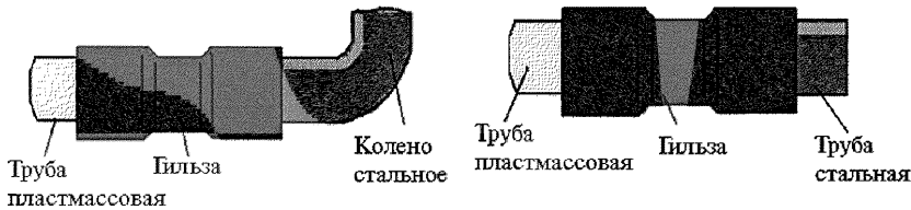
Рисунок 5.49 – Соединение пластмассовых труб при скрытой прокладке
