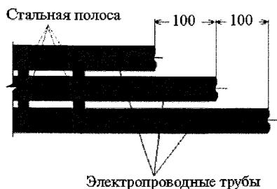
Рисунок 5.41 – Размещение электропроводных труб в блоке соединяемых труб
