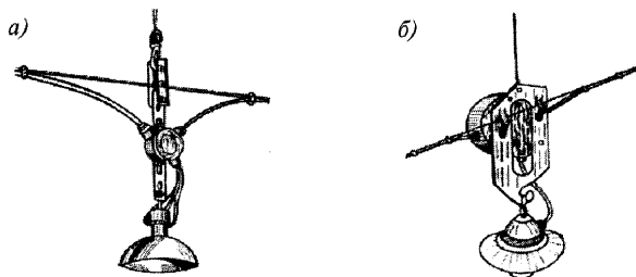
Рисунок 5.30 – Пример подвески и подключения светильника при выполнении тросовых электропроводок
