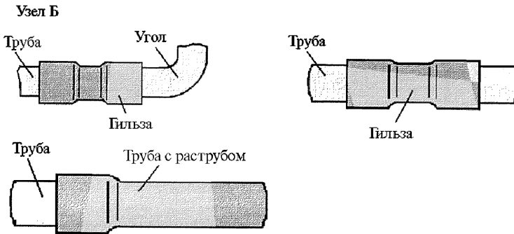
Рисунок 5.46 – Открытая прокладка пластмассовых труб
