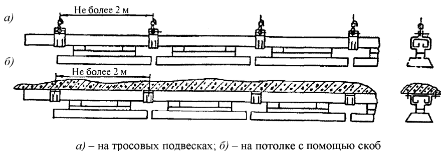
Рисунок 5.9 – Крепление металлических коробов со светильниками с люминесцентными лампами
