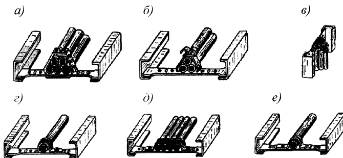
а) – крепление кабелей к лоткам с помощью ленты с кнопкой; б), в) – крепление кабелей к лоткам с помощью полоски-пряжки; г), д), з) – крепление кабелей к лоткам с помощью скобы;
