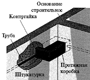
Рисунок 5.40 – Переход труб с одной стены на другую
