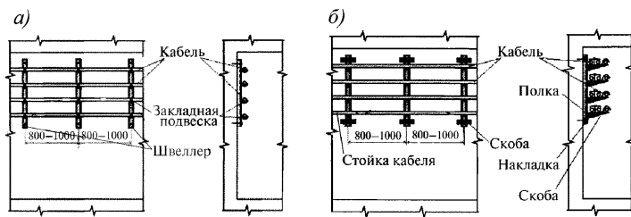
а) – на подвесках; б) – на полках
