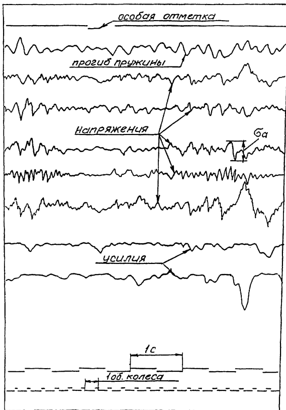
Рисунок 5 - Образец осциллограммы
