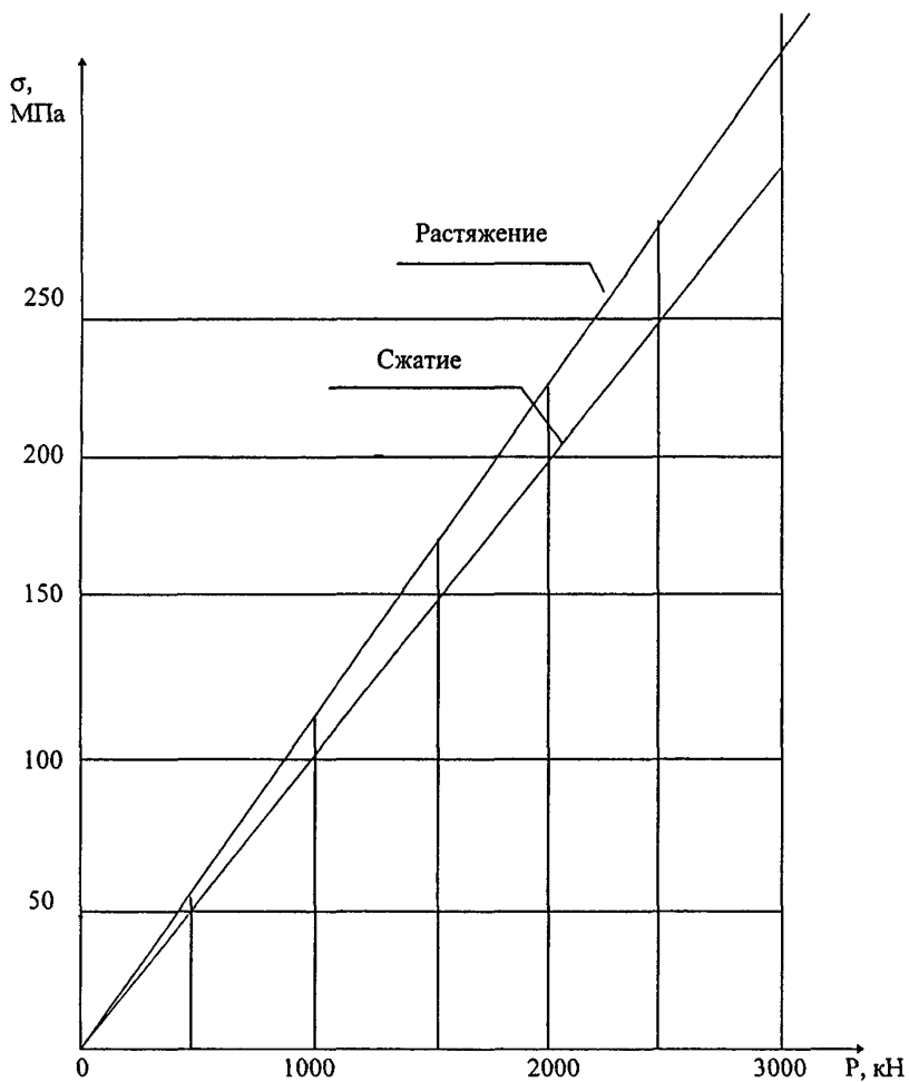
Рисунок 1 - График градуировки автосцепки
