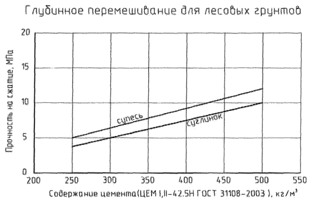
Рисунок Ф.3 – Зависимость прочности грунтоцемента от содержания цемента в 1 м³ ГЦЭ
