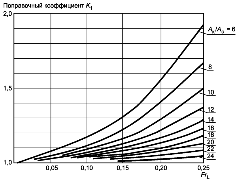
Рисунок 8.3 — Номограмма для определения поправочного коэффициента K_1 для канала неполного профиля по числу Фруда Fr_L и отношению площадей A_k/A_c
