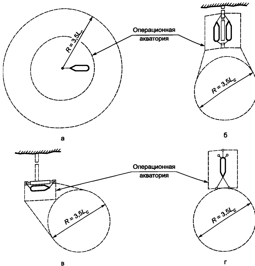
а — для одностоечных причалов и зон ожидания на стоянке, а также для причалов типа «выносное причальное устройство», б и в — для островных причалов, г — для многостоечных причалов
