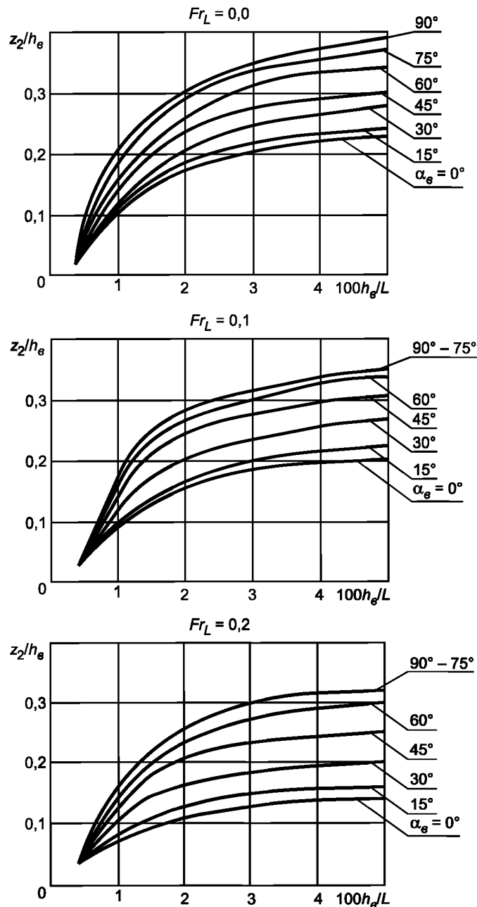
Рисунок 8.1 — Номограмма для определения отношения запаса от волновых воздействий к высоте волны z_2/h_e , при различных углах волнения \alpha_e и числах Фруда Fr_L
