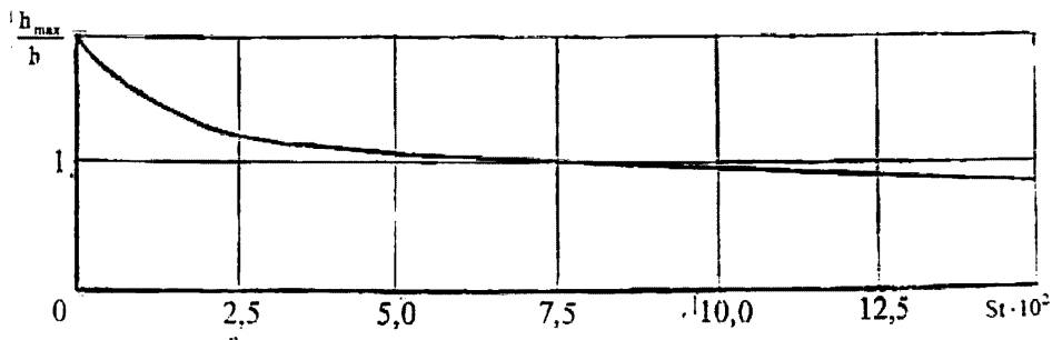
Рисунок Г.3 – График для определения высоты волны на уресе
