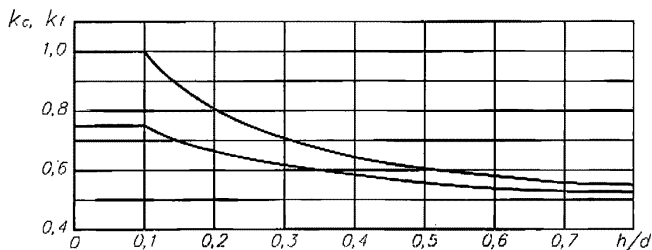
Рисунок 7.1 – Графики значений коэффициентов k_c , k_f
