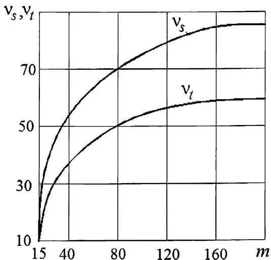
Рисунок 6.8 – Зависимость отношения v_s, v_t от уклона берега
