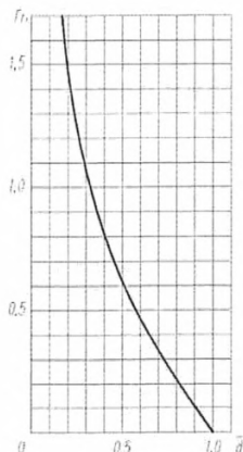
Рисунок 8.4 – График для определения величины Fr_1
