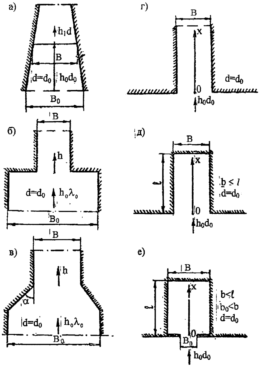
Рисунок Д.2 – К определению высоты воли при изменении геометрических размеров акваторий
