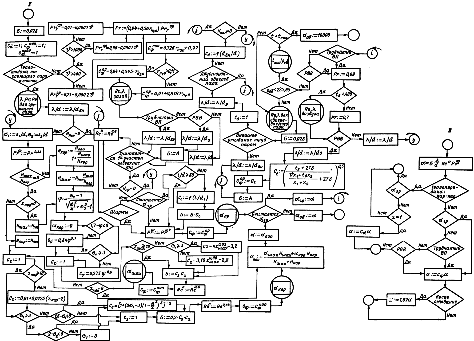
I — определение \alpha_k для рассчитываемой поверхности нагрева; II — общая схема расчета коэффициента теплоотдачи конвекцией
