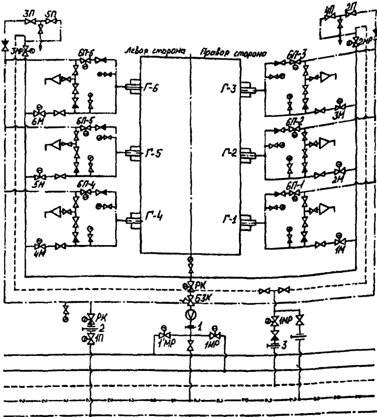
Рис. 2. Схема паромазутопроводов водогрейного котла КВГМ-180-150:
