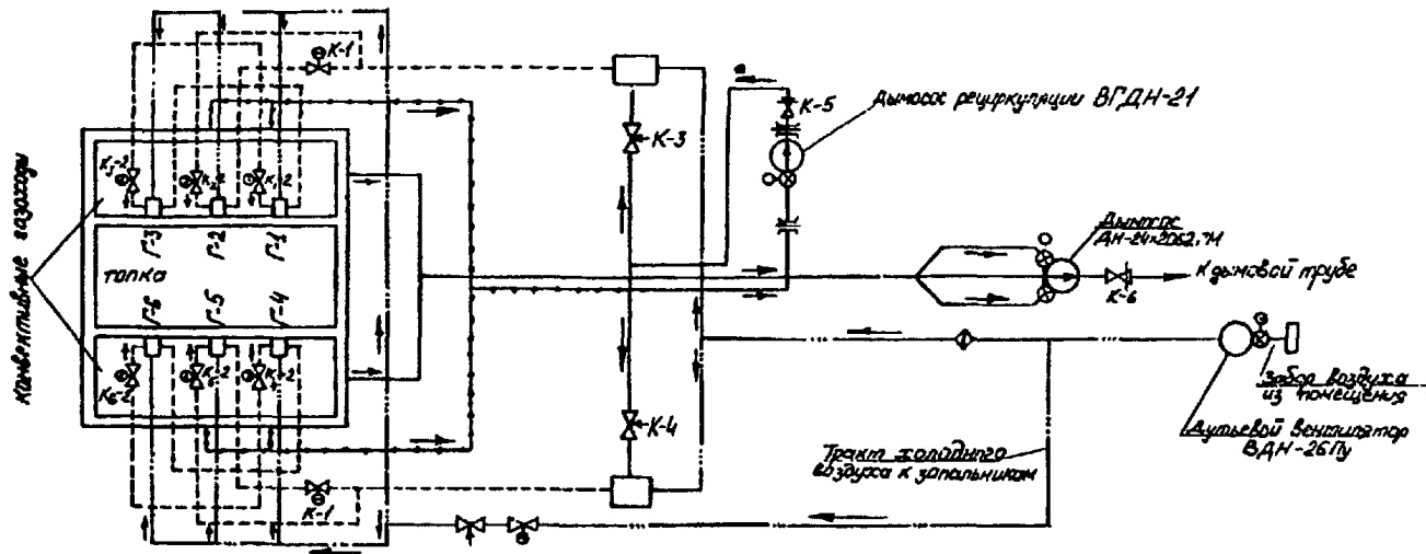
Рис. 1. Схема газозухопроводов водогрейного котла КВГМ-180-150:
