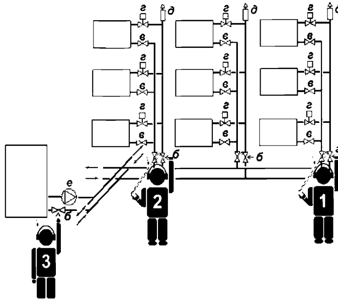
a – эталонный клапан балансировочный; б – клапаны-партнеры балансировочные; в – запорно-регулирующий клапан; z – термостатический клапан; д – воздухоотводчик; e – насос
