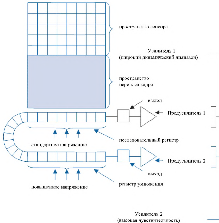
Рис. 12 Структура EM-CCD матрицы
