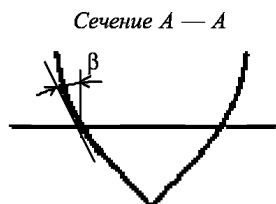
Угол наклона шпангоута \beta
