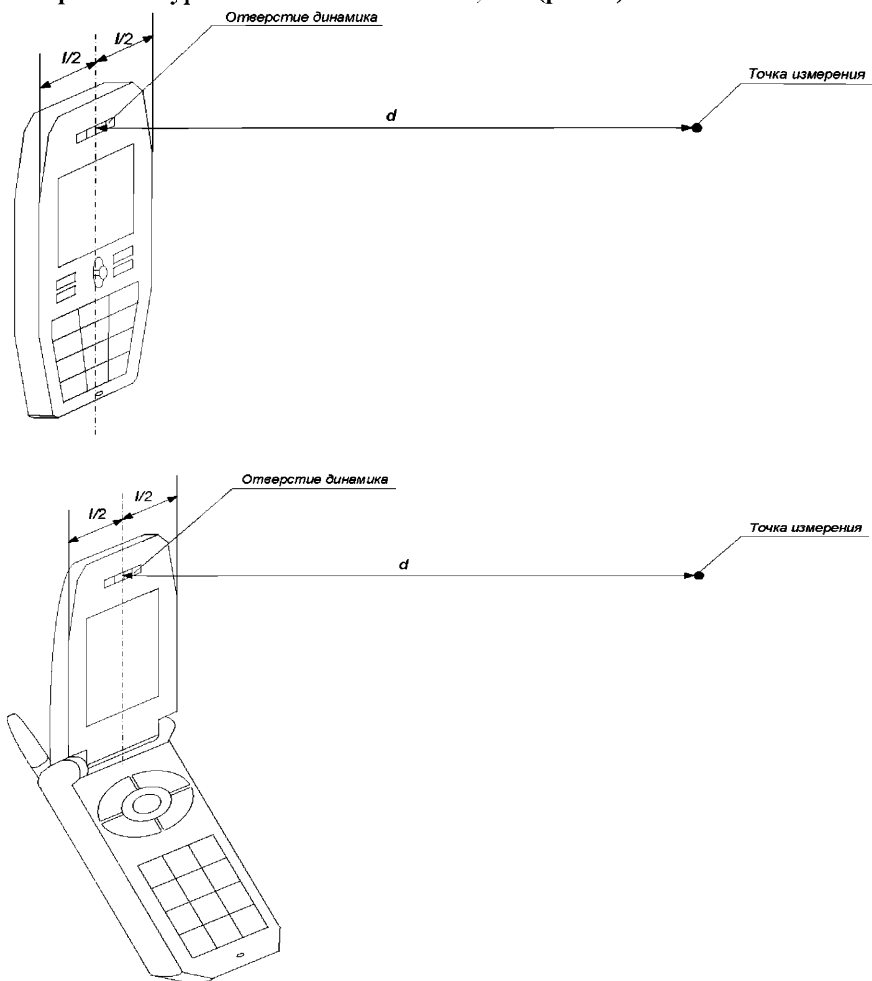
Рис. 1. Точка измерений интенсивности ЭМП РЧ, создаваемого АТ различной конструкции
