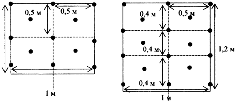
Рис. 2. Примеры выделения точек измерения на контролируемых поверхностях элементов стационарных защитных устройств защитной камеры
