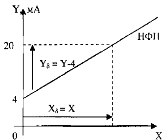
Рисунок 2а – Подавление нуля выходного сигнала, например датчика
