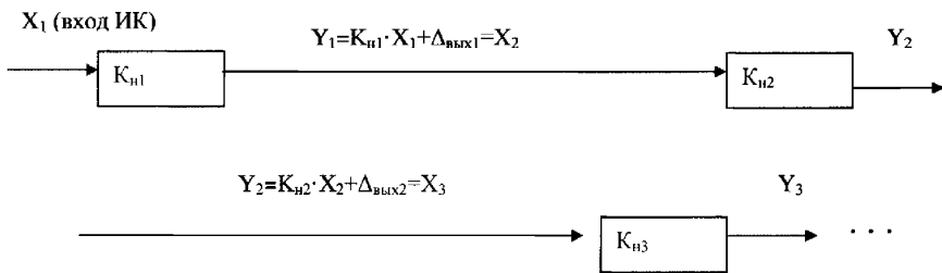
Рисунок 3 – «Накопление» погрешностей в простом ИК
