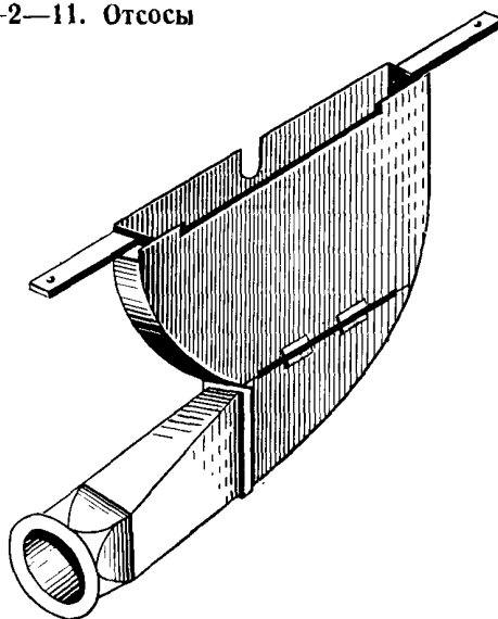
Рис. 26. Отсос от циркульной пилы
