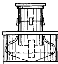
Рис. 15. Дефлектор типа ЦАГИ.
