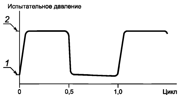
Рисунок F.1 — Цикл импульса давления
