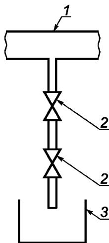
Рисунок 10 — Пробоотборник в виде трубопровода с двойным краном
