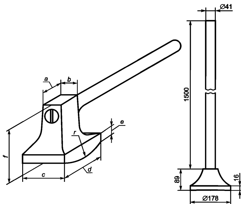
Рисунок 4 — Типичный молоток для дробления крупных частиц (кусков)
