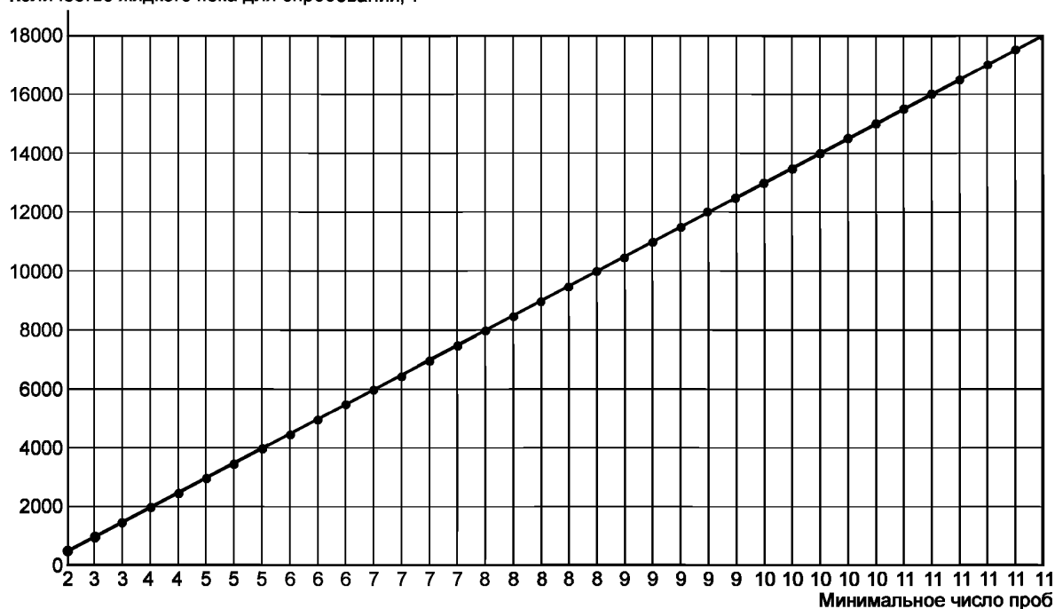
Рисунок 6 — Количество проб жидкого пека в зависимости от количества пека, качество которого определяют
