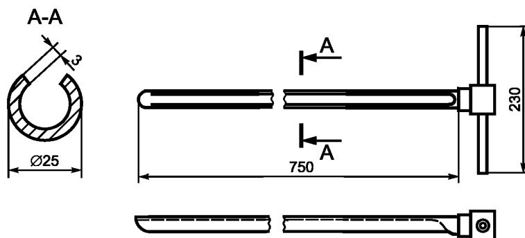
Рисунок 3 — Пробоотборник закрытого типа — типичные размеры
