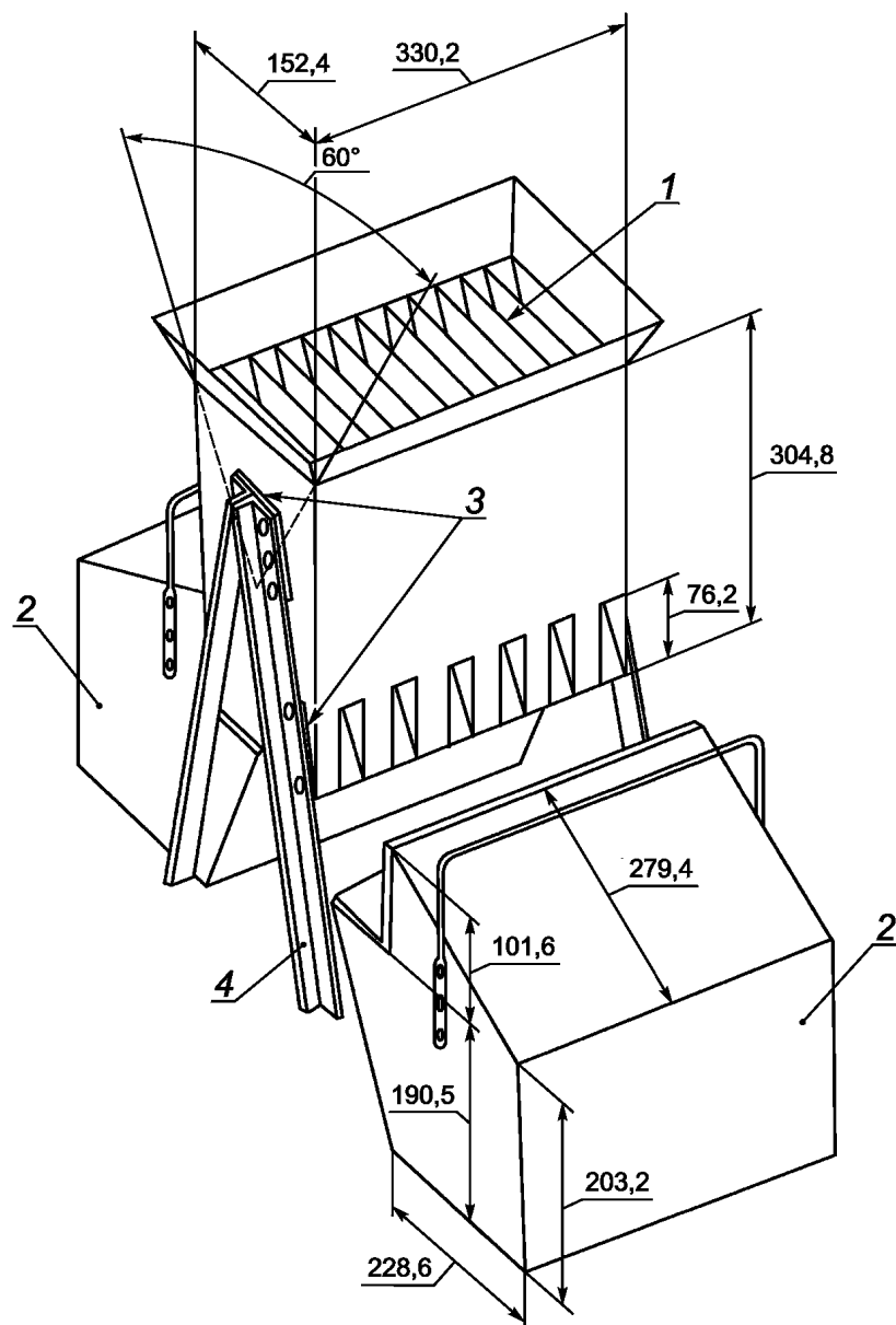
1 — двенадцать желобов размером (25,4 мм); 2 — приемник; 3 — прокладки на кронштейнах (12,7 мм) для обеспечения просвета для контейнера; 4 — угловые кронштейны размером (25,4 мм)
