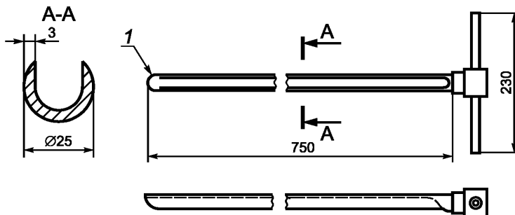
Рисунок 2 — Пробоотборник открытого типа — типичные размеры
