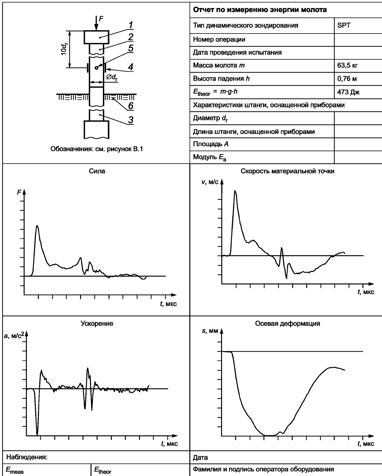
Рисунок В.2 — Пример отчета об измерениях энергии молота
