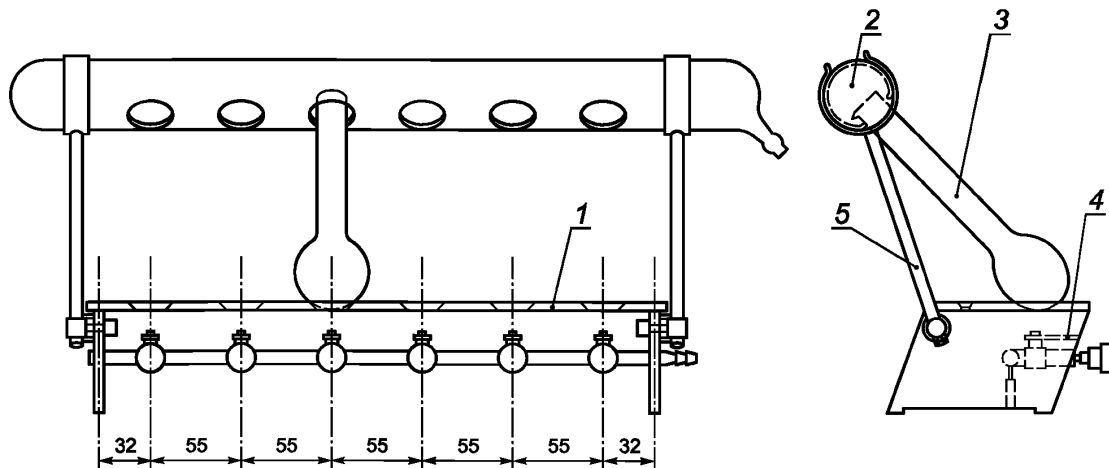
1 — полка из термостойкого теплоизоляционного материала; 2 — выпускная трубка; 3 — колба для кипячения; 4 — микрорегелка; 5 — опорный стержень с регулировкой угла наклона и длины
