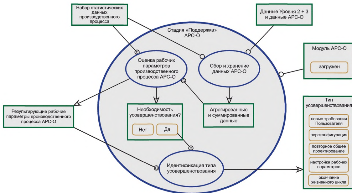
Рисунок 5 — Рабочий процесс стадии «технической поддержки»
