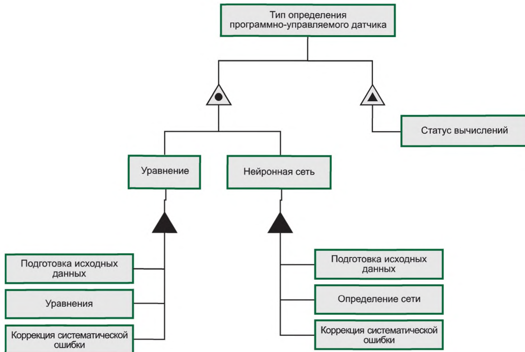
Рисунок 20 — Пример типа определения программно-управляемого датчика SoftSensor
