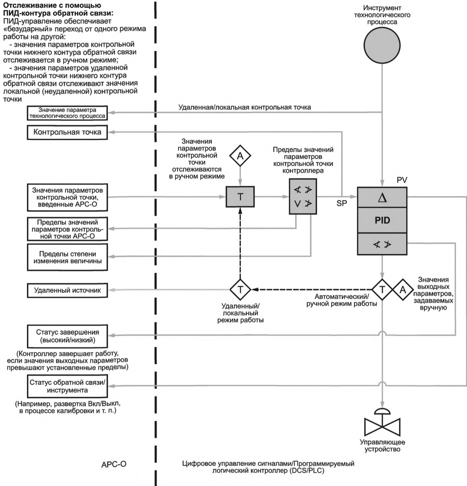
Рисунок 10 — Взаимодействие APC-O с традиционным ПИД-контуром обратной связи
