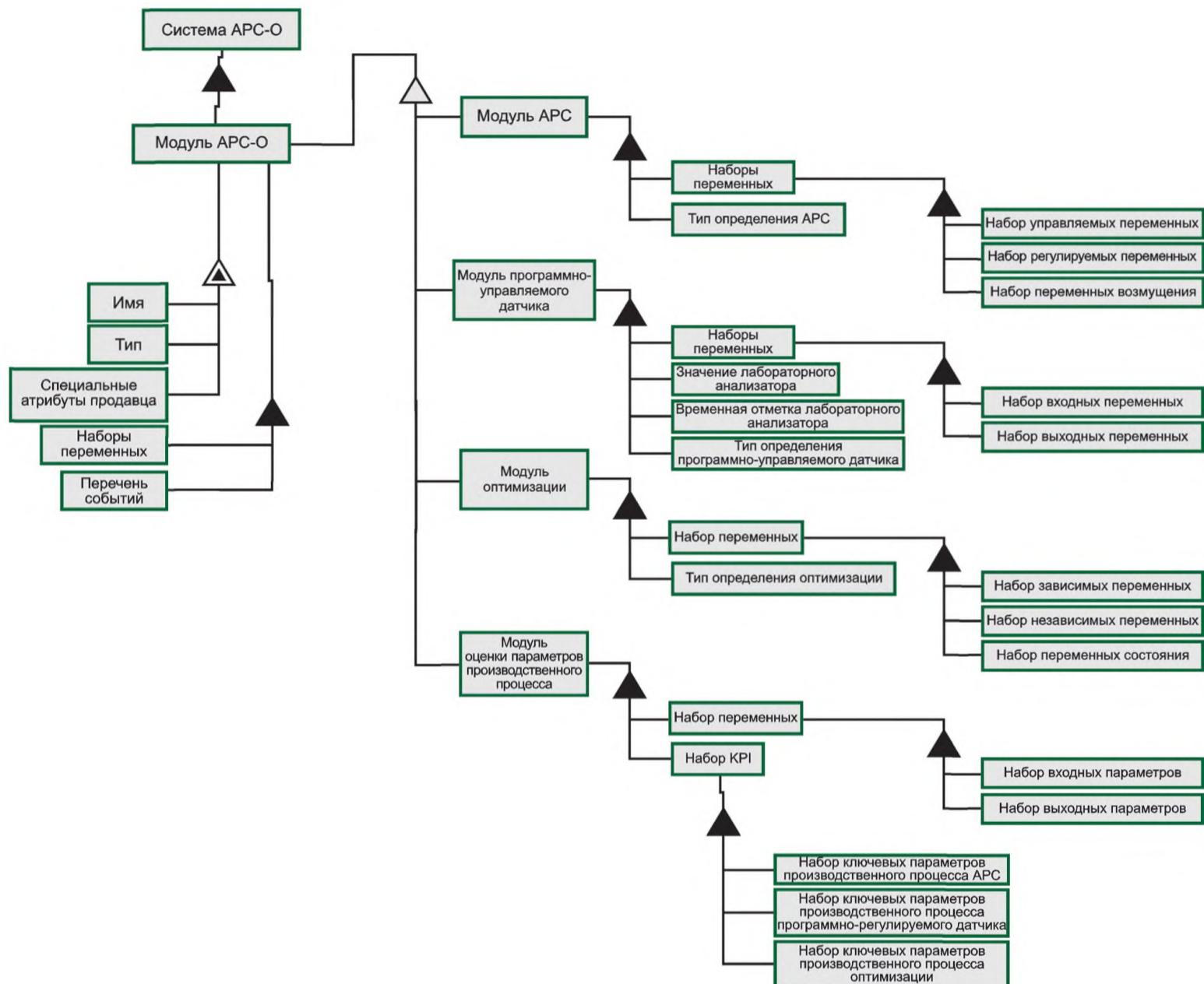
Рисунок 6 — Информационная модель APC-O
