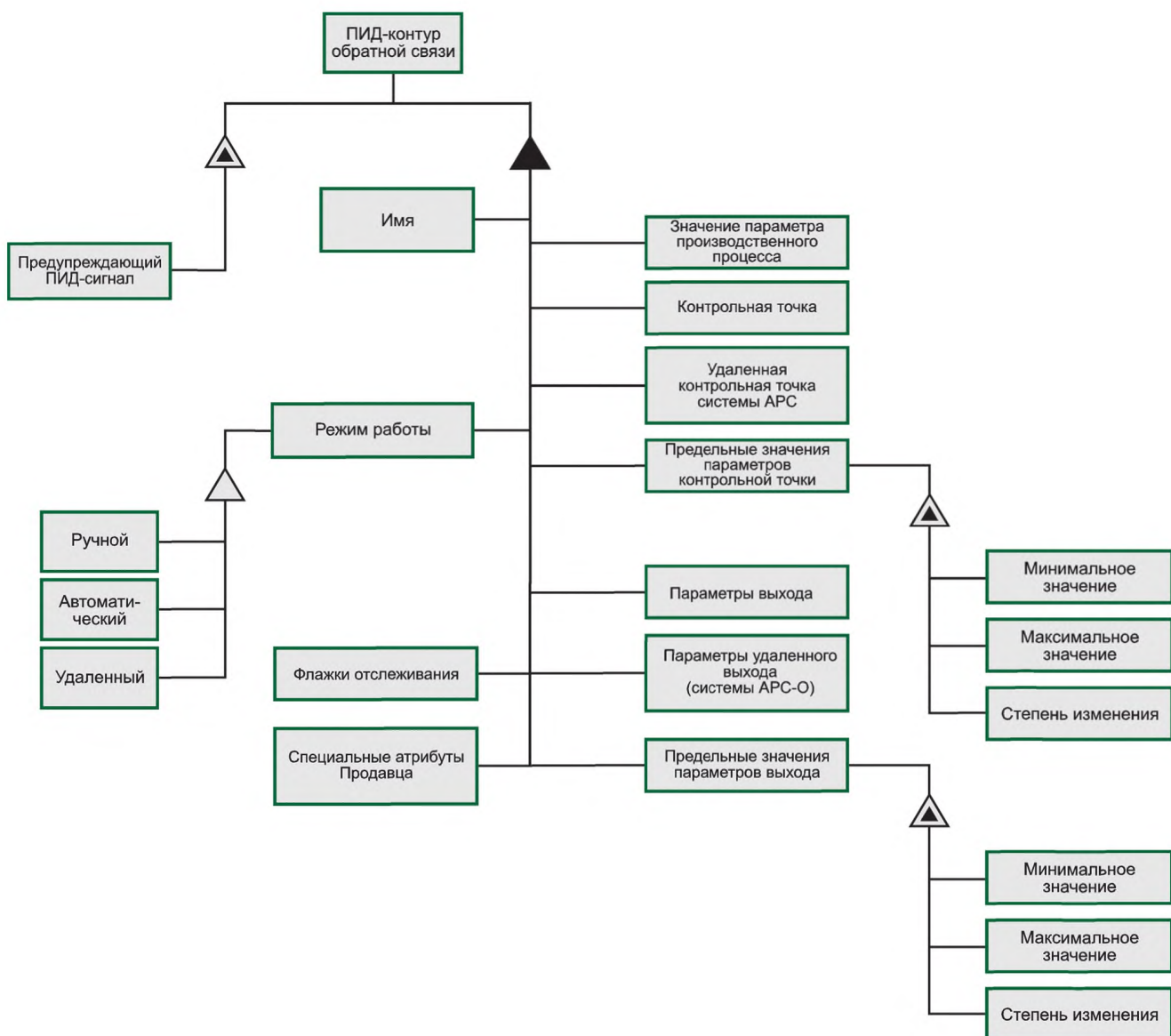
Рисунок 9 — Информационная модель ПИД-контура обратной связи PIDLoop
