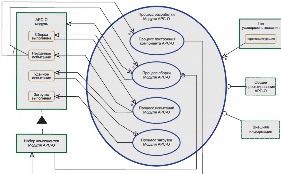
Рисунок 2 — Рабочий процесс на стадии «разработка»
