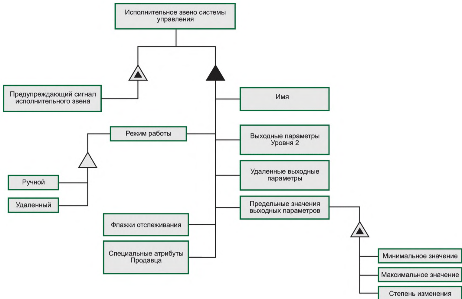
Рисунок 11 — Информационная модель исполнительного звена системы управления FinalControlElement
