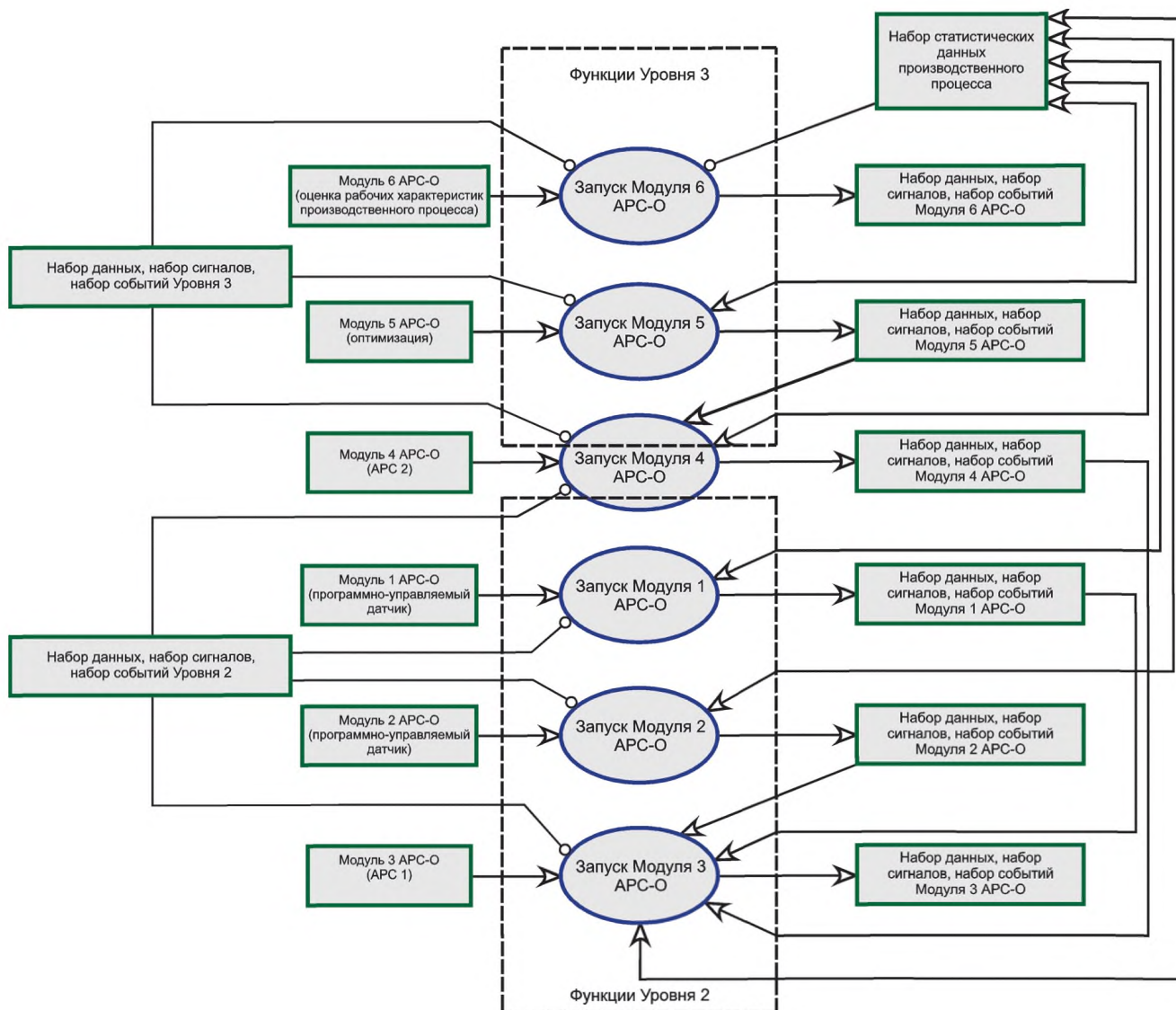
Рисунок 4 — Пример распределенного взаимодействия APC-O компонентов
