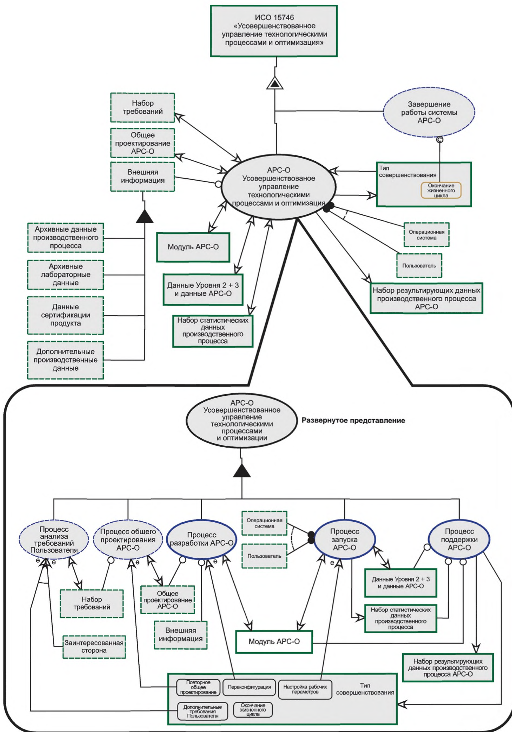
Рисунок 1 — Рабочий процесс жизненного цикла APC-O модуля
