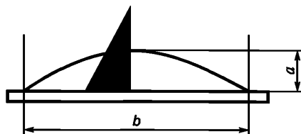
Рисунок 3 — Пример 1 общего диагонального перекоса
