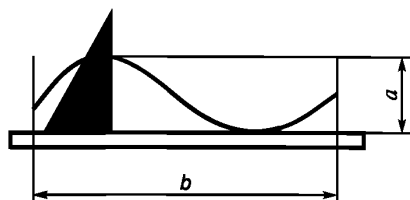
Рисунок 5 — Пример 3 общего диагонального перекоса
