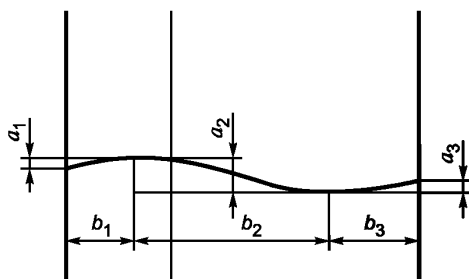
Рисунок 8 — Местный диагональный перекос (модель по трем треугольникам)
