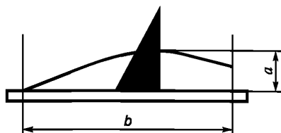
Рисунок 4 — Пример 2 общего диагонального перекоса
