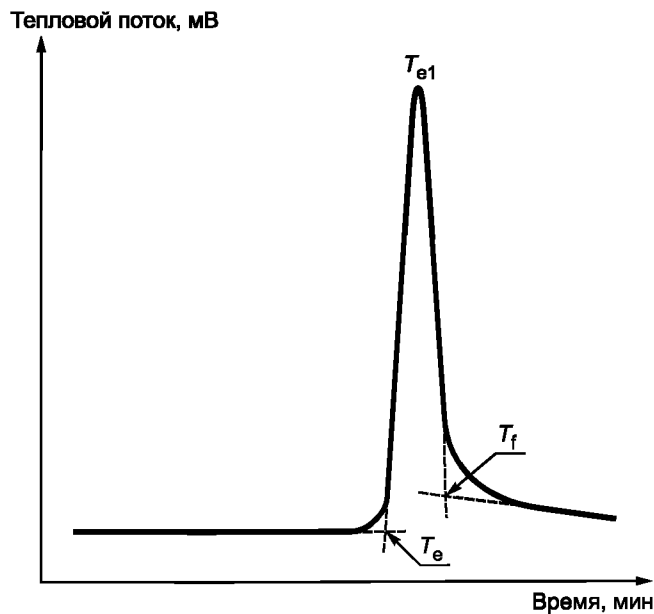
Рисунок 2 — ДСК-кривая охлаждения
