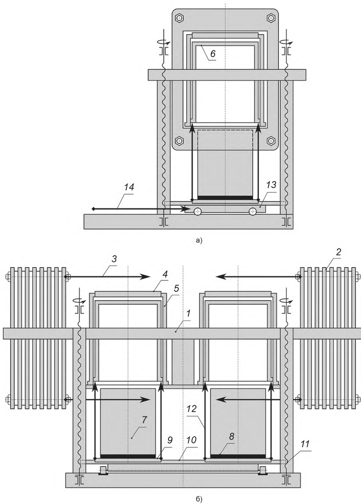
Рисунок 2 — Кинематическая схема силового модуля: а) вид сбоку; б) вид фронтальный (позиции обозначения — в соответствии с таблицей 2)
