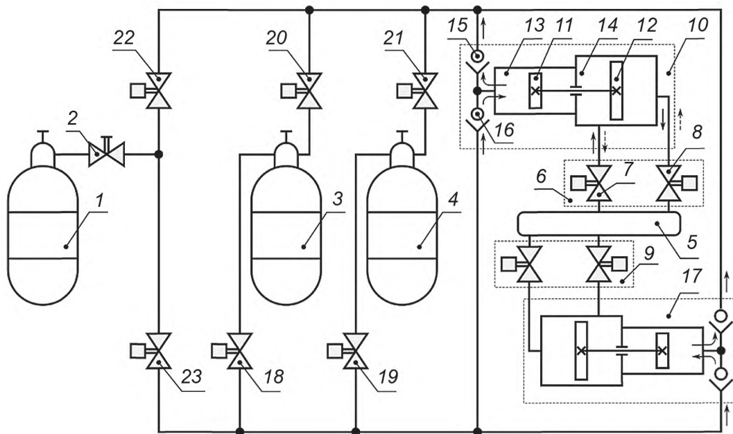
Рисунок 3 — Пневмогидравлическая схема газокompрессорной системы агрегата УКС
