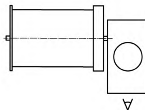
б) лебедка правого исполнения с односекционным барабаном
