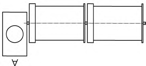
в) лебедка левого исполнения с двухсекционным барабаном
