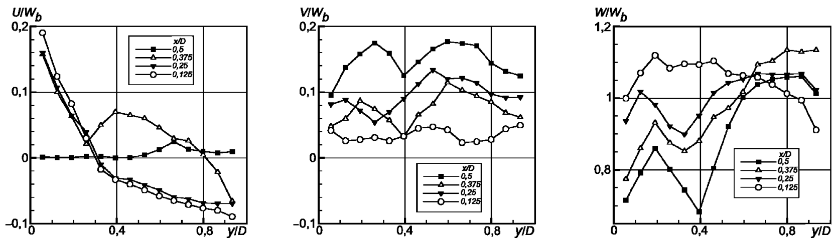
Рисунок 6 — Три компоненты скорости в сечении \psi = \pi/2
