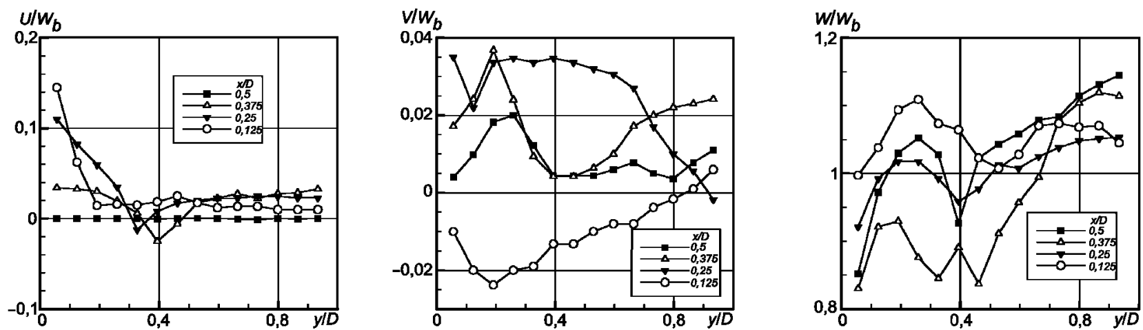
Рисунок 8 — Три компоненты скорости в сечении \psi = 3\pi/4
