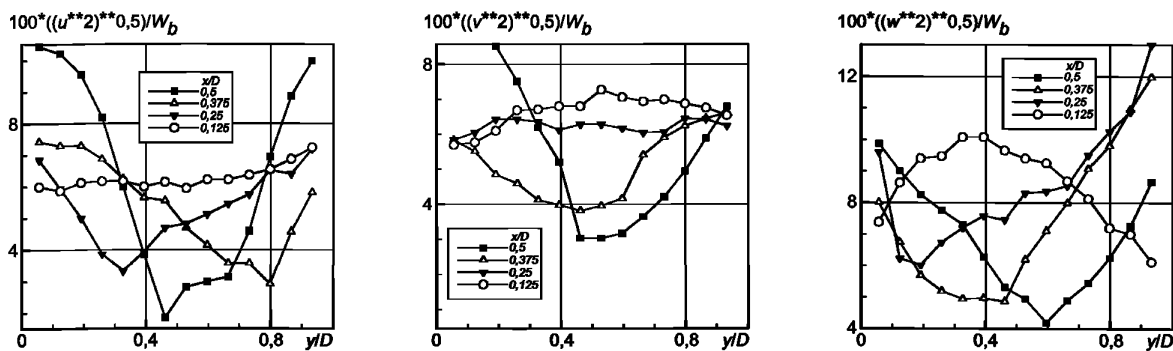
Рисунок 3 — Нормальные компоненты напряжений Рейнольдса в сечении \psi = 0
