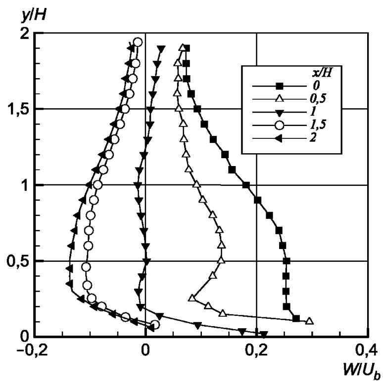
Рисунок 46 — Боковая компонента скорости в плоскости z/H = 1
