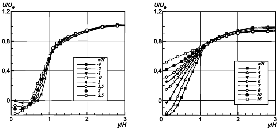
Рисунок 28 — Продольная компонента средней скорости
