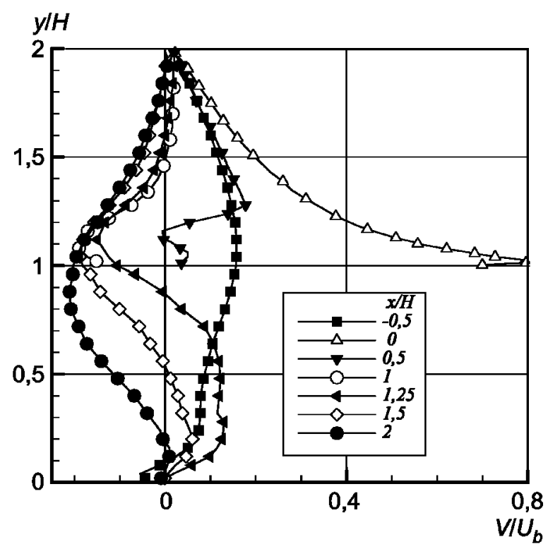
Рисунок 42 — Вертикальная компонента скорости в плоскости z/H = 0,5
