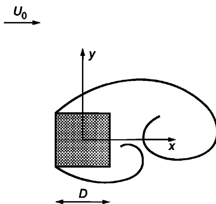
Рисунок 54 — Турбулентная дорожка Кармана за квадратным цилиндром
