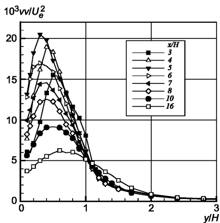
Рисунок 31 — Нормальные напряжения Рейнольдса в поперечном направлении
