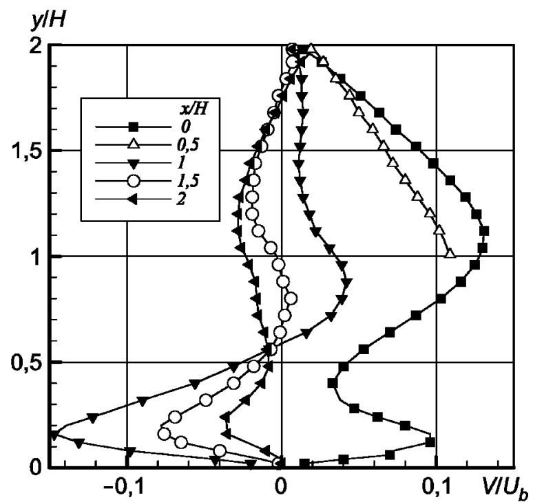
Рисунок 45 — Вертикальная компонента скорости в плоскости z/H = 1
