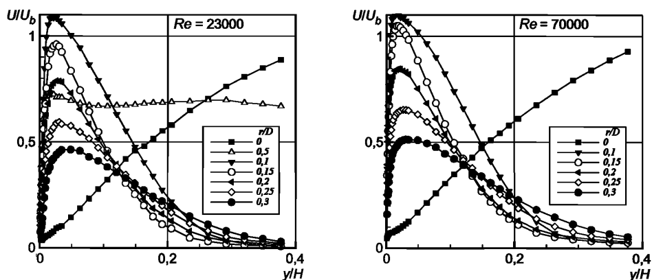
Рисунок 23 — Продольная компонента скорости
