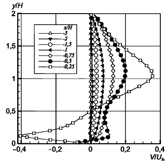
Рисунок 38 — Вертикальная компонента скорости перед препятствием в плоскости z/H = 0
