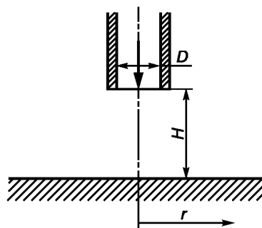
Рисунок 22 — Круглая струя, нормально падающая на плоскость
