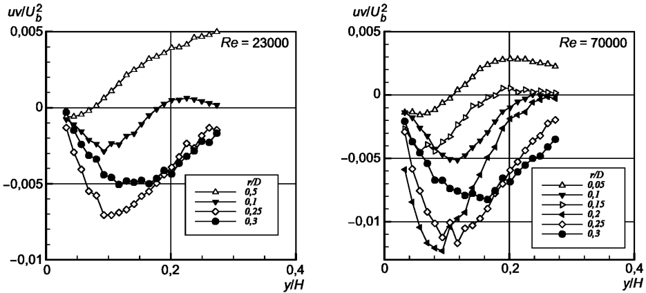
Рисунок 26 — Сдвиговые напряжения Рейнольдса
