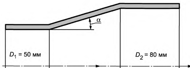
Рисунок 47 — Течение в конически расширяющейся трубе
