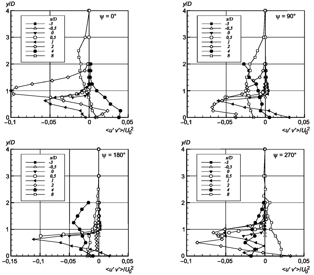
Рисунок 59 — Профили сдвиговых напряжений Рейнольдса
