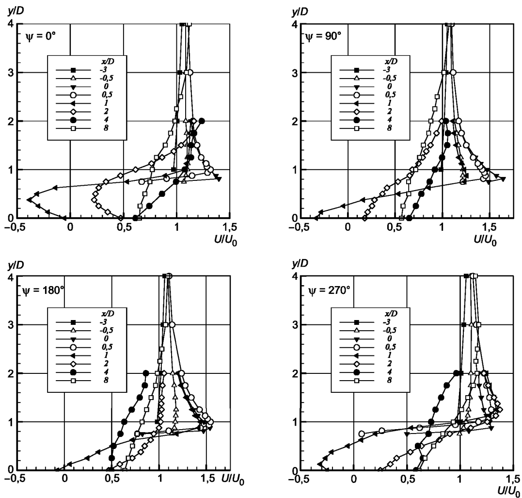
Рисунок 55 — Профили продольной компоненты средней скорости
