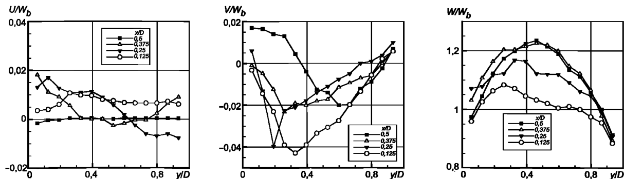
Рисунок 2 — Три компоненты скорости в сечении \psi = 0
