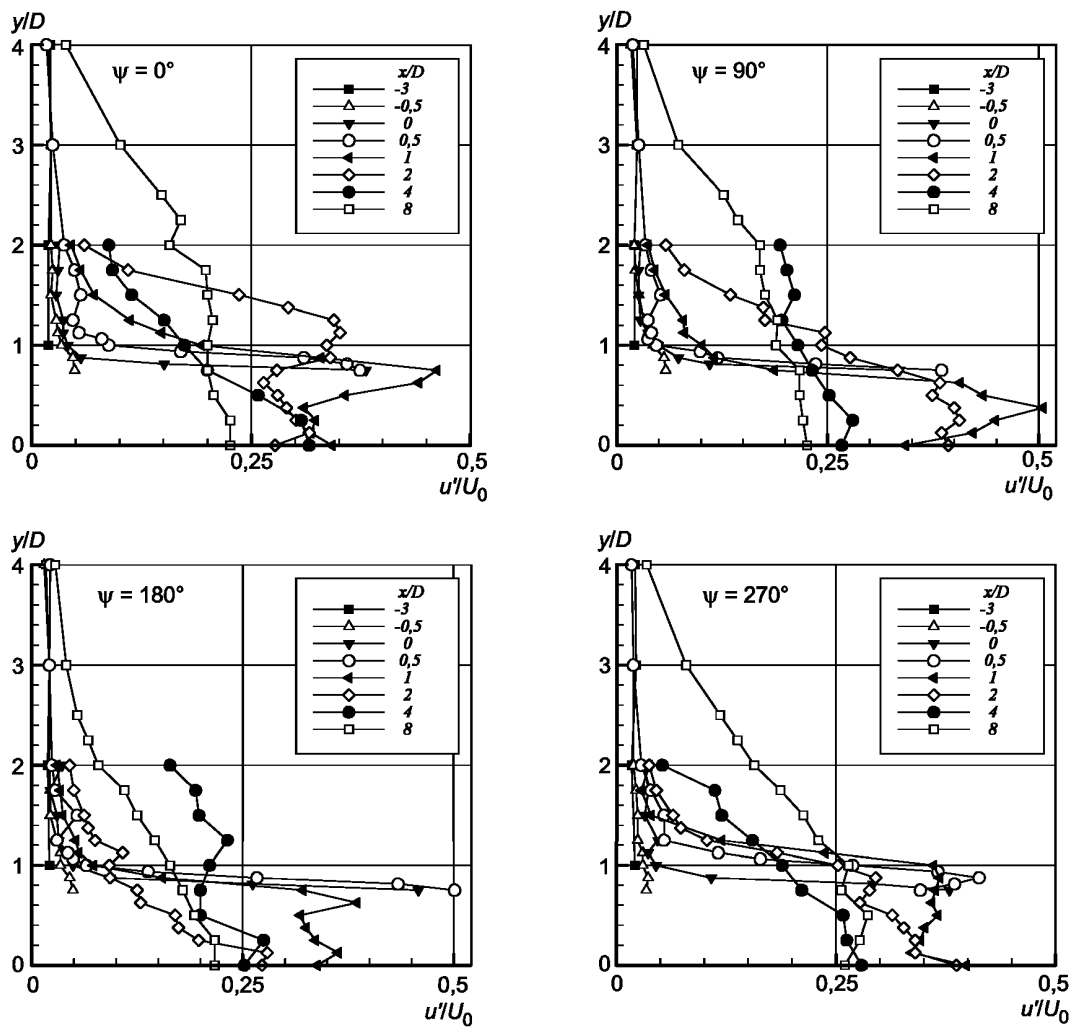
Рисунок 57 — Профили интенсивностей пульсаций скорости в продольном направлении
