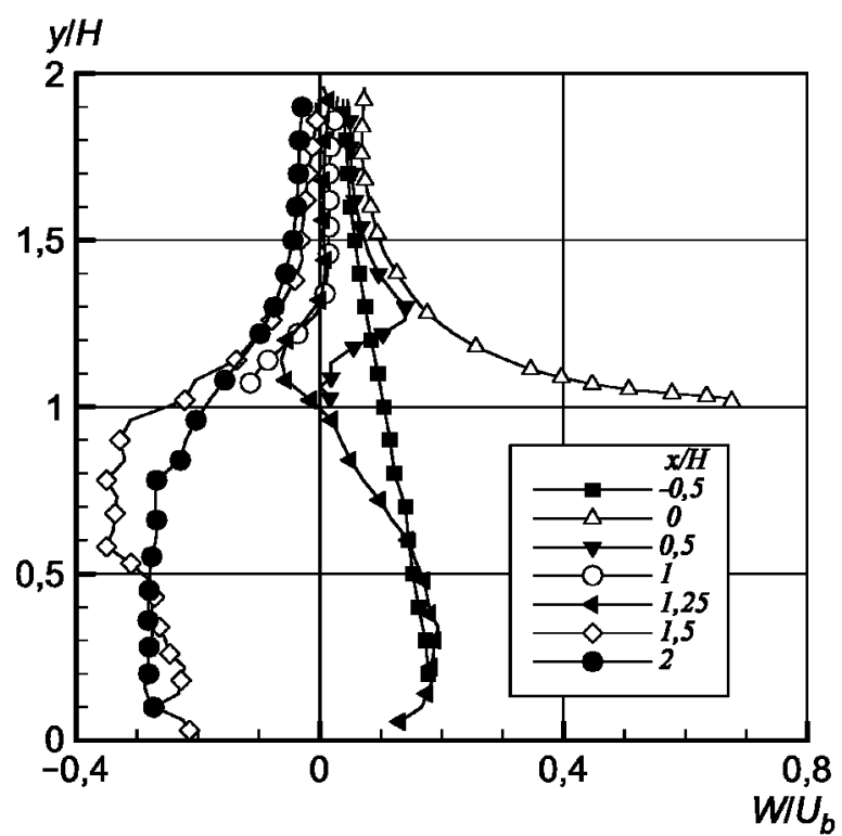
Рисунок 43 — Боковая компонента скорости в плоскости z/H = 0,5
