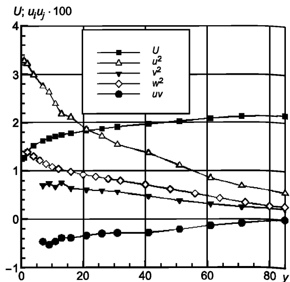
Рисунок 19 — Профиль скорости U (м/с) и профили компонент напряжений Рейнольдса u_i u_j ( \text{м}^2/\text{с}^2 ) в набегающем потоке. Координата y в мм
