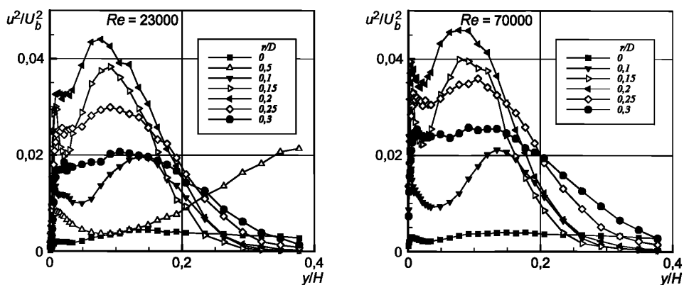
Рисунок 24 — Нормальные напряжения Рейнольдса
