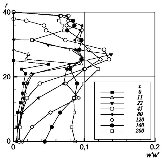
Рисунок 52 — Нормальные напряжения Рейнольдса в угловом направлении; x и r в мм, w'w'' в \text{м}^2/\text{с}^2
