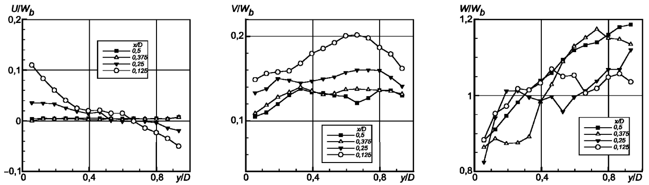
Рисунок 10 — Три компоненты скорости в сечении \psi = \pi
