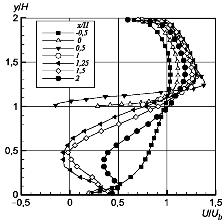
Рисунок 41 — Продольная компонента скорости в плоскости z/H = 0,5
