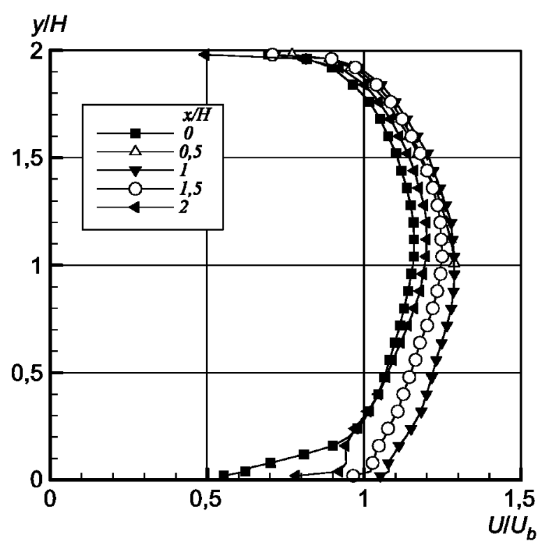
Рисунок 44 — Продольная компонента скорости в плоскости z/H = 1
