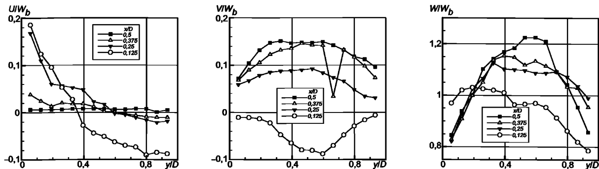
Рисунок 4 — Три компоненты скорости в сечении \psi = \pi/4
