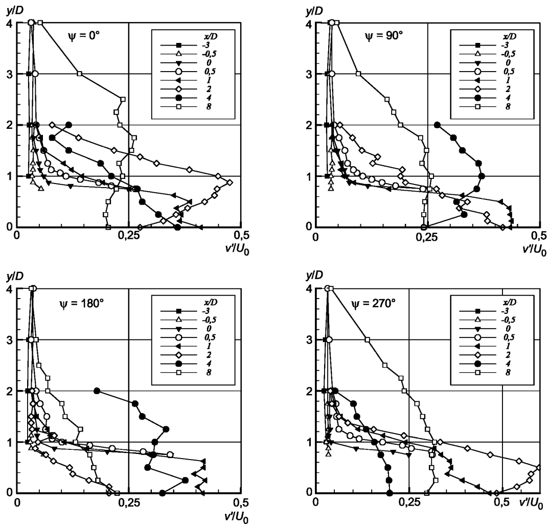
Рисунок 58 — Профили интенсивностей пульсаций скорости в поперечном направлении
