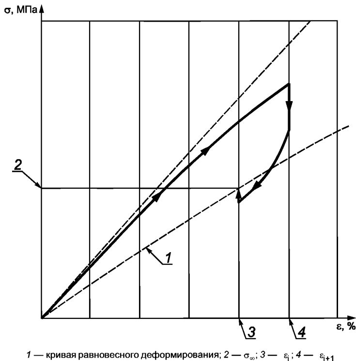
Рисунок 1 — Схема эксперимента по определению равновесного значения напряжения \sigma_\infty при заданной деформации \varepsilon
