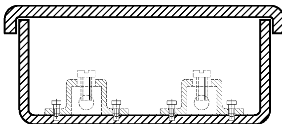
c — с условиями для вставки впоследствии окончных или соединительных устройств
