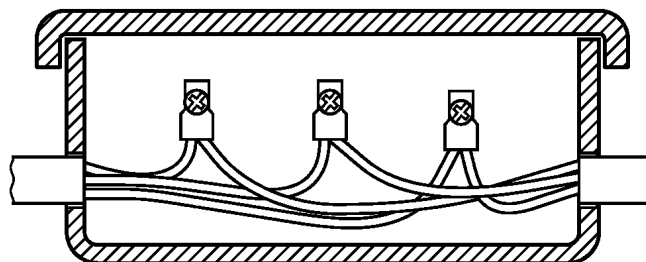
d — с плавающими окончными или соединительными устройствами
