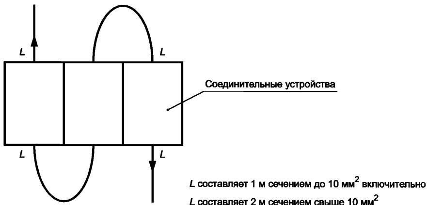
Рисунок 102 — Многопозиционное оконечное устройство
