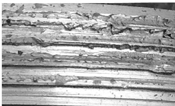
б) Рванины на витках наружной резьбы
