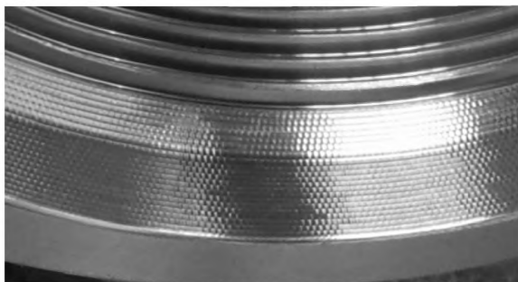
б) Следы вибрации, приводящие к несоответствию геометрических параметров расточки и заходной фаски
