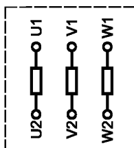
Рисунок 3 — Трехфазное электрооборудование с шестью выводами
