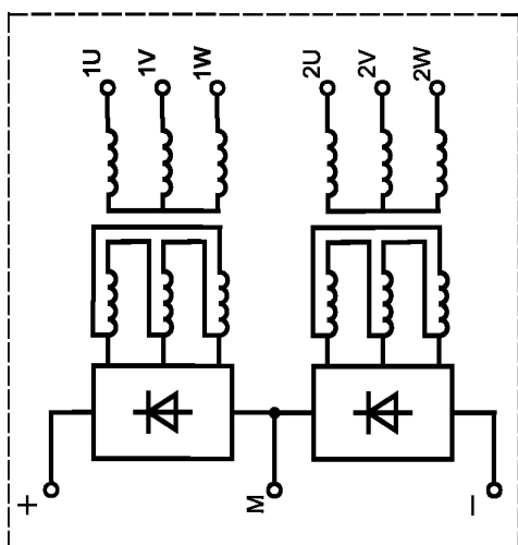
Рисунок 5а — Трехфазное электрооборудование с двумя группами элементов
