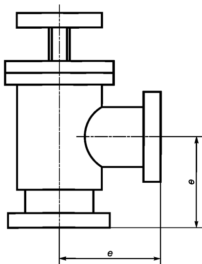
Рисунок 1 — Установочные размеры вакуумных соединений углового клапана
