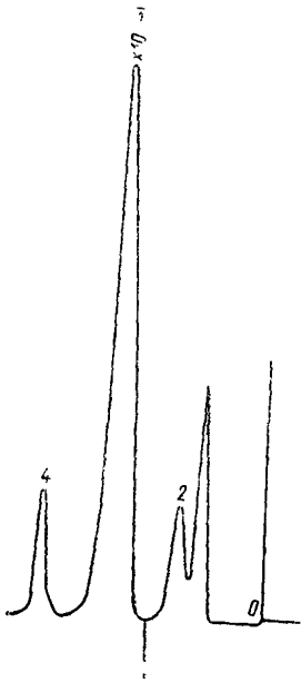
Типовая хроматограмма бромистого этила
