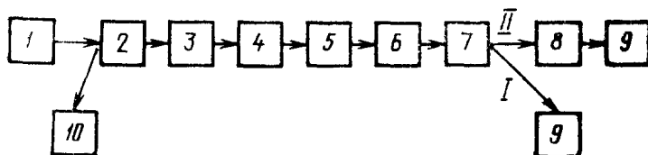
Схема установки для измерения коэффициента преобразования ЭОП в динамическом режиме
