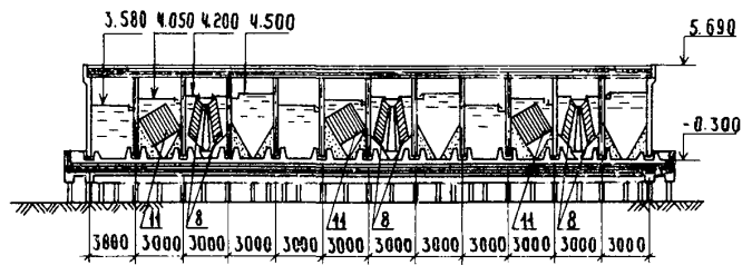
РАЗРЕЗ I-I
