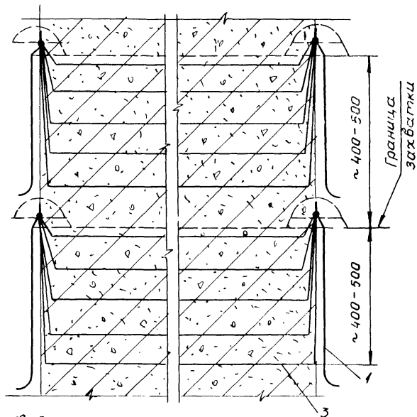
Схема подключения нагревательных проводов к магистральным отводам
