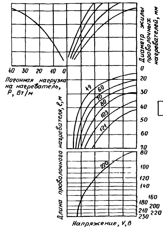
Рис. 3. Номограмма для определения длины проволочных нагревателей
