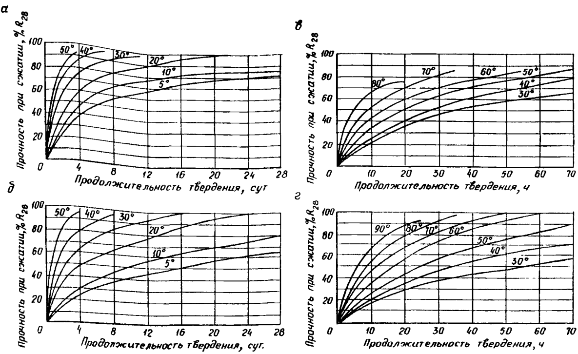
Рис. 5. Кривые набора прочности бетоном при различных температурах его выдерживания:
