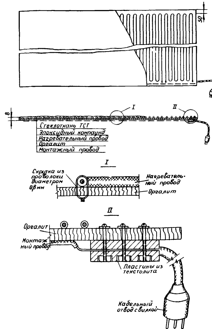
Рис. 1. Грейный плоский элемент (ГЭП)
