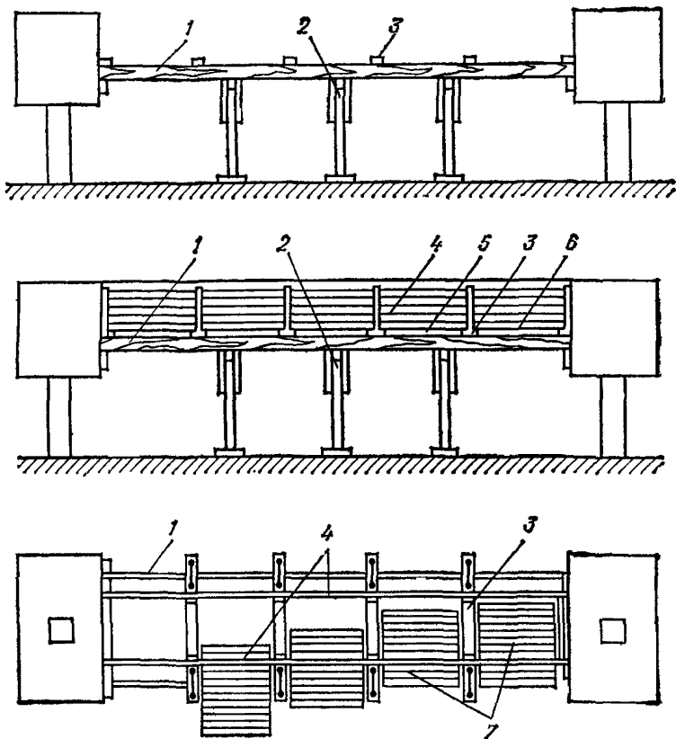
Рис. 65. Последовательность операций по устройству опалубки для снеговывдувающей конструкции бетонирования ростверковых систем
