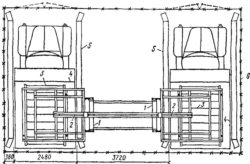
Рис. 15. Схема площадки для электронагрева бетонной смеси в кузовах автосамосвалов
