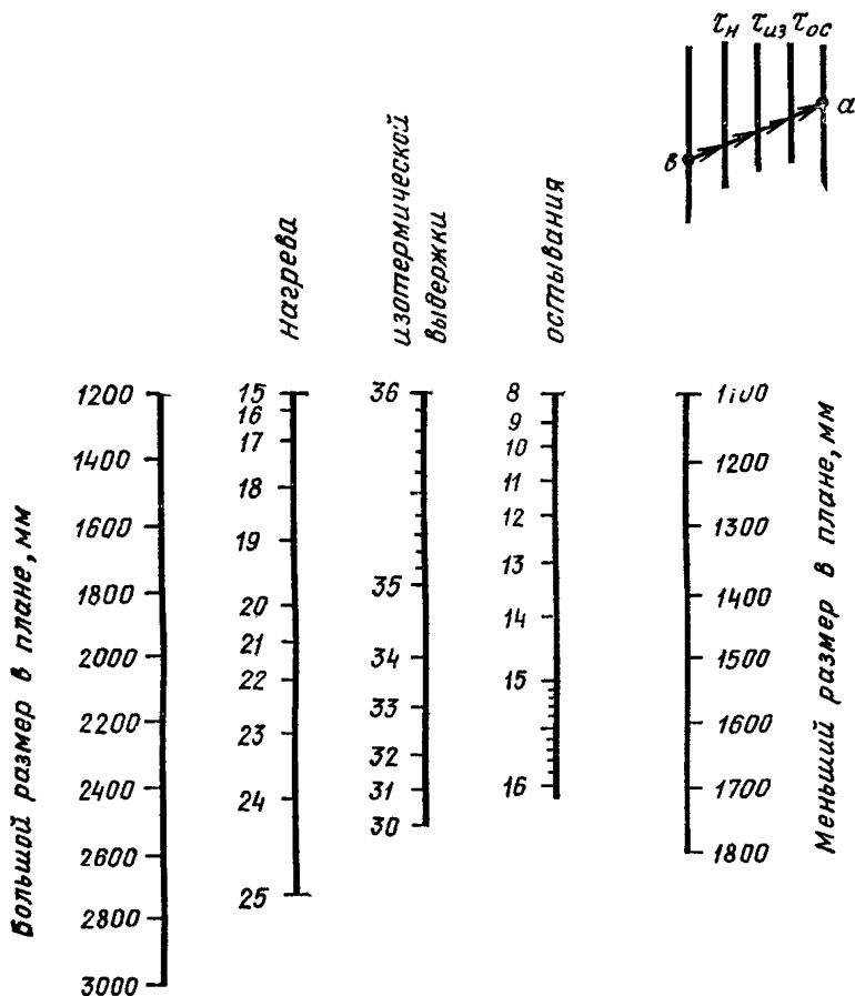
б — номограмма для определения продолжительности термообработки монолитных массивных фундаментов столбчатого типа высотой более 1 м;
