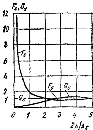
Рис. 53. Зависимость безразмерных коэффициентов сопротивления F_s и Q_s для металлической плиты (листа) от относительной толщины
