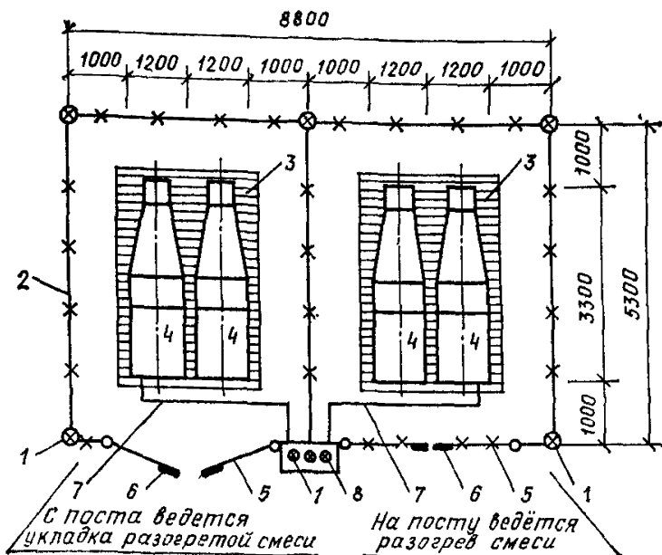
Рис. 14. Схема площадки электронагрева бетонной смеси в бункерах
