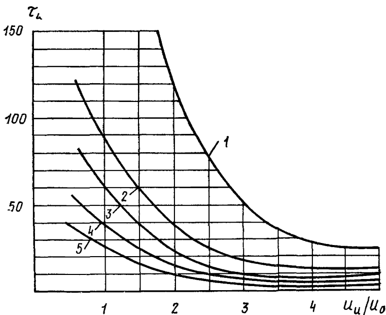
Рис. 31. График определения продолжительности импульсов тока при импульсном прогреве
