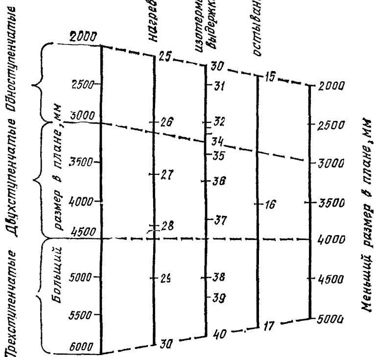
2 — номограмма для определения продолжительности термообработки монолитных ступенчатых фундаментов с высотой ступеней 500 мм
