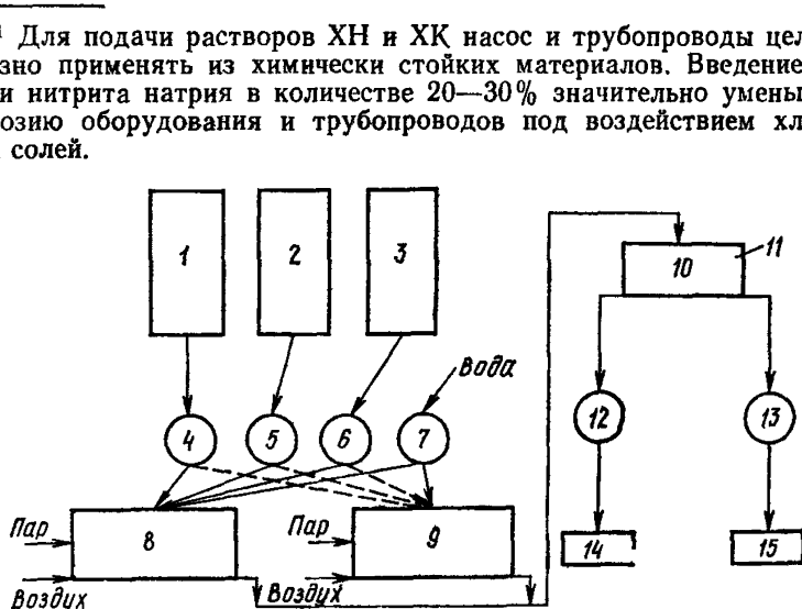
Рис. 78. Схема технологического процесса при предварительном приготовлении раствора добавки рабочей концентрации
