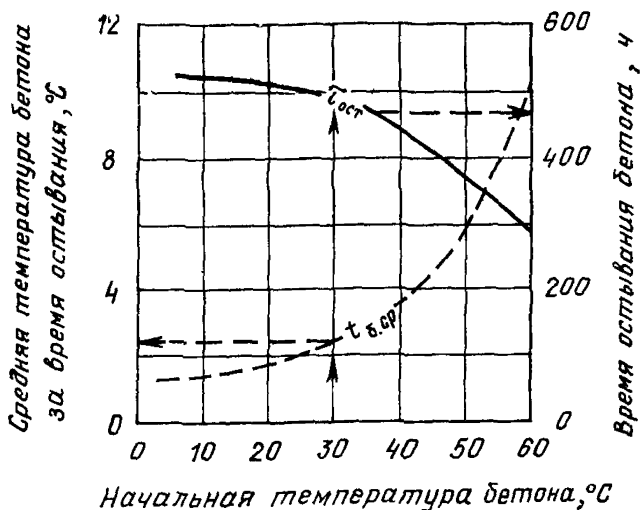
Рис. 9. Время остывания бетона до 0° С ( t_{\text{ост}} ) и средняя температура бетона ( t_{\text{б.ср.}} ) за это время в зависимости от начальной температуры бетона
