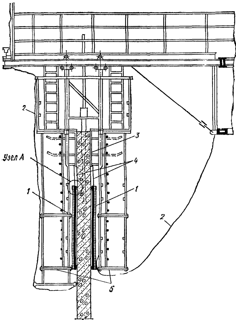
Рис. 51. Схема возведения трубы с применением термоактивных подвесных покрытий 1 — ТАПП; 2 — брезентовое укрытие; 3 — скользящая опалубка; 4 — подвеска ТАПП; 5 — подвесные леса
