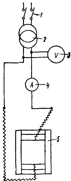
Рис. 81. Схема определения удельного сопротивления бетона
