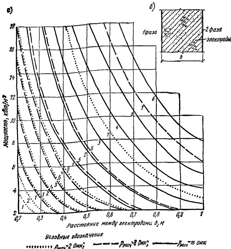
Рис. 18. Электропрогрев бетона пластинчатыми электродами а — график для расчета при напряжении на электродах; б — схема подключения; 1, 2, 3, 4, 5, 6, 7 — при напряжении соответственно 49, 60, 70, 85, 103, 121 и 220 В
