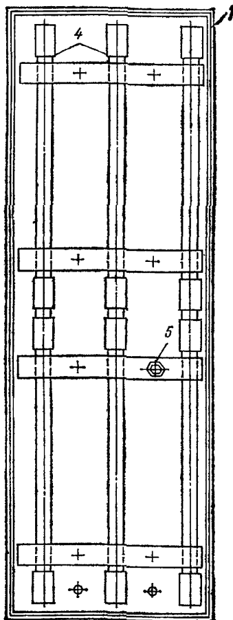
Рис. 63. Схема термовкладыша греющей опалубки стыков 1 — каркас уголков; 2 — панель из электроизоляционного материала; 3 — ТЭНы; 4 — утеплитель; 5 — болты для крепления термовкладыша к щиту опалубки; 6 — защитный кожух
