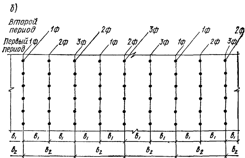
Рис. 30. Изменение схемы коммутации электродов для выдерживания заданного температурного режима в разные периоды прогрева а — полосовые электроды при периферийном прогреве; б — стержневые электроды
