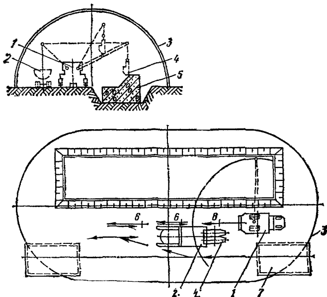
Рис. 59. Механизированная укладка бетонной смеси в тепляке с использованием схемы «кран — бадья»
