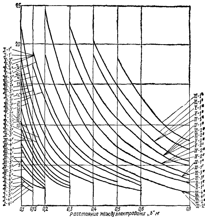
Рис. 206. График для расчета периферийного прогрева при одностороннем расположении полосовых электродов бетона конструкций толщиной B=20 см (обозначения по рис. 20 в)
