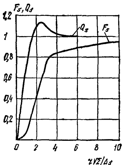
Рис. 54. Зависимость безразмерных коэффициентов сопротивления для металлического стержня от аргумента
