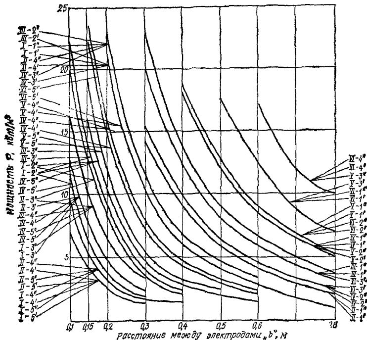
Рис. 20а. График для расчета периферийного прогрева при одностороннем расположении полосовых электродов бетона конструкций толщиной B=10 см (обозначения по рис. 20 в)
