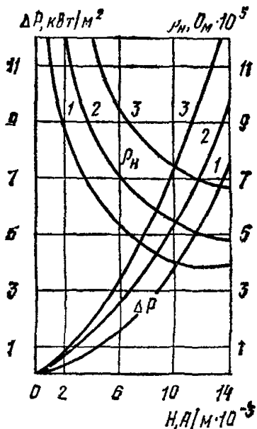
Рис. 52. Зависимость удельного поверхностного электросопротивления \rho_n и удельной активной мощности \Delta P от напряженности магнитного поля H
