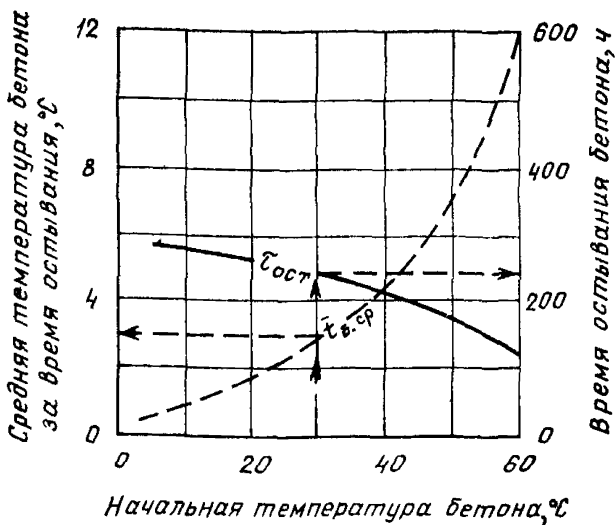
Рис. 7. Время остывания бетона до 0^{\circ}\text{C} ( \tau_{\text{ост}} ) и средняя температура бетона ( t_{\text{б.ср}} ) за это время в зависимости от начальной температуры бетона
