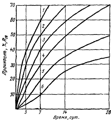
Рис. 76. Нарастание прочности бетона с добавкой НН при 10°С (1), 5°С (2), 0°С (3), -5°С (4), -10°С (5) и -15°С (6)
