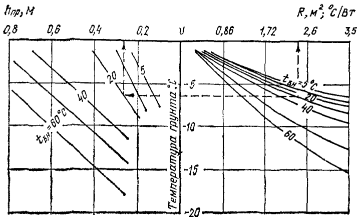
Рис. 8. График для определения параметров бетонирования монолитной плиты на мерзлом песчаном основании с влажностью 5% при наборе бетоном прочности до замерзания 70% R_{28} ( t_{\text{б.н}} — начальная температура бетона)
