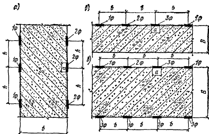
Рис. 19. Схемы размещения и подключения полосовых электродов a — при сквозном прогреве; б — при одностороннем периферийном прогреве конструкций толщиной 30 см; в — при периферийном прогреве конструкций толщиной более 30 см
