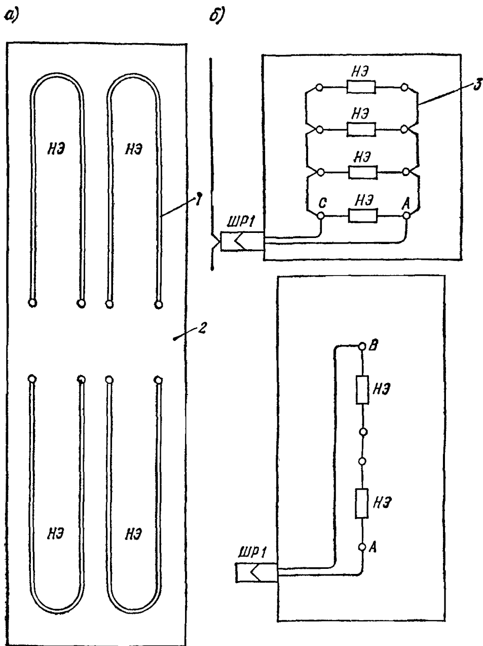
Рис. 74. Пример схемы монтажа и расположения нагревательных элементов a — размещение нагревателей, б — параллельная и последовательная схемы соединения нагревателей; 1 — ТЭНы; 2 — панель из электроизоляционного материала
