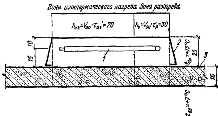
Рис. 83. Схема к расчету параметров инфракрасной установки для обогрева стены, возводимой в скользящей опалубке
