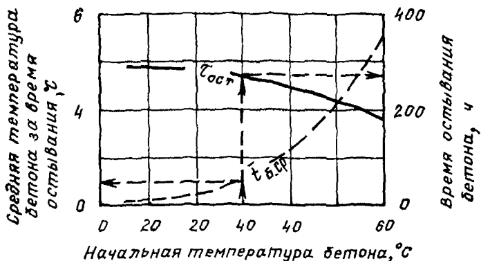
Рис. 11. Время остывания бетона до 0^{\circ}\text{C} ( \tau_{\text{ост}} ) и средняя температура бетона ( t_{\text{б.ср}} ) за это время в зависимости от начальной температуры бетона
