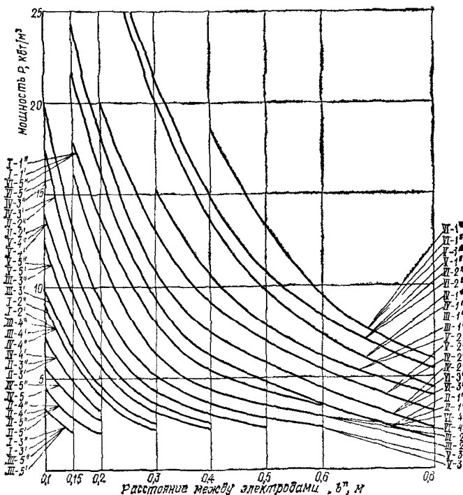
Рис. 20в. График для расчета периферийного прогрева при одностороннем расположении полосовых электродов бетона конструкций толщиной B=30 см I-1, I-2, I-3, I-4, I-5 — при напряжении 49 В; II-1, II-2, II-3, II-4, II-5 — 60 В; III-1, III-2, III-3, III-4, III-5 — 70 В; IV-1, IV-2, IV-3, IV-4, IV-5 — 85 В; V-1, V-2, V-3, V-4, V-5 — 103 В; VI-1, VI-2, VI-3, VI-4, VI-5 — 121 В; расчетное удельное электрическое сопротивление 1, 2, 3, 4, 5 — соответственно 2, 4, 8, 12, 16 Ом·м; при ширине полосовых электродов 0,02 м — 1', 2', 3', 4', 5' и 0,05 м — 1'', 2'', 3'', 4'', 5''
