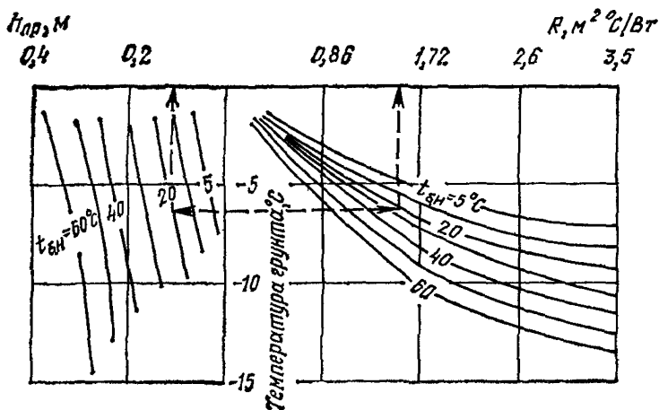
Рис. 10. График для определения параметров бетонирования монолитной плиты на мерзлом песчаном основании с влажностью 10% при наборе бетоном прочности до заморозания 50% R_{2\%} ( t_{\text{б.н.}} — начальная температура бетона после укладки)
