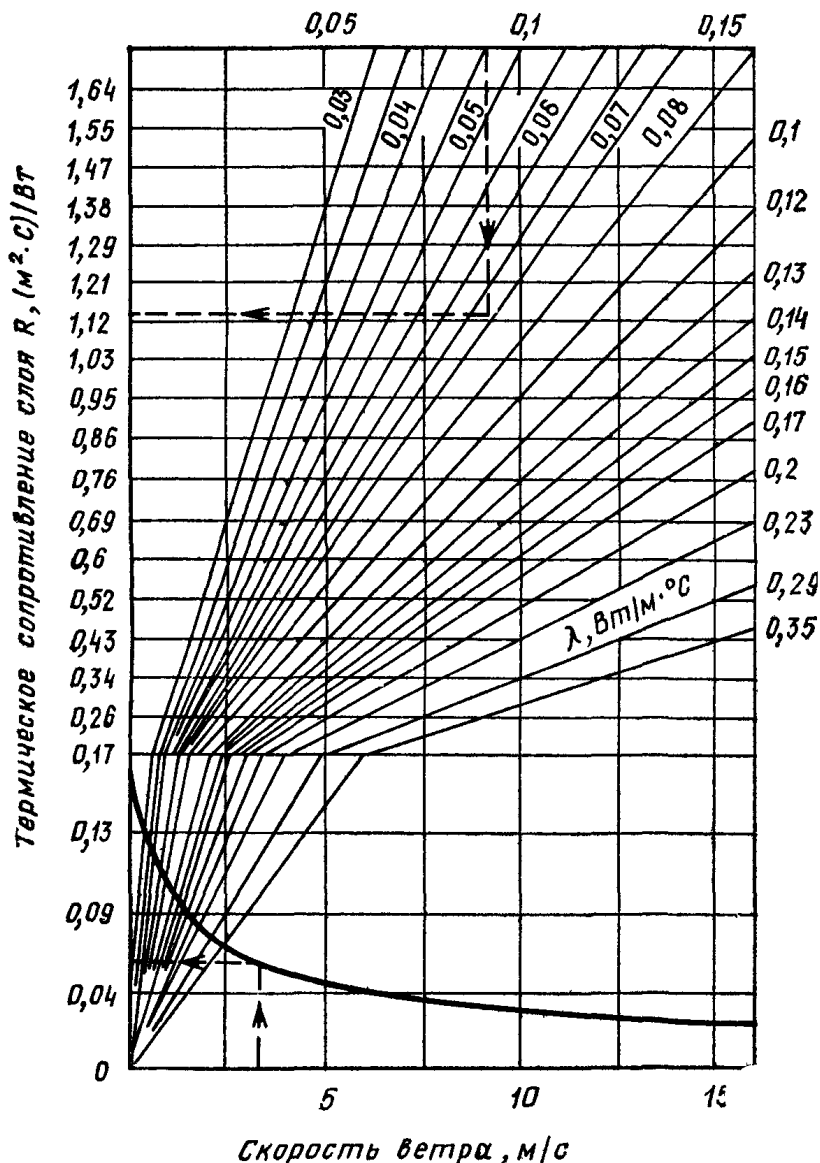
Рис. 5. Номограмма для определения термического сопротивления опалубки в зависимости от скорости ветра и термических сопротивлений слоев опалубки
