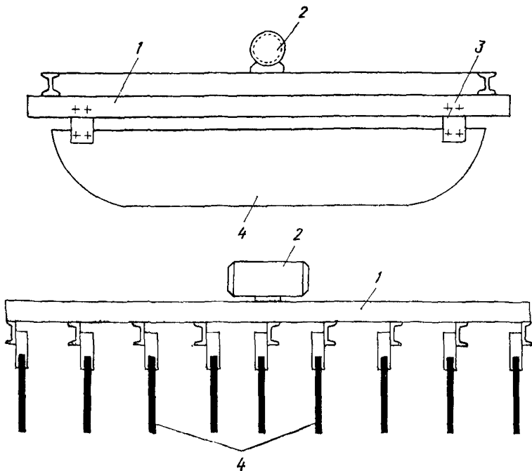
Рис. 13. Принципиальная схема опускающего устройства для электроразогрева бетонной смеси в кузовах автосамосвала 1 — рама; 2 — вибратор; 3 — электроизолированные крепления электродов; 4 — пластинчатые крепления электродов
