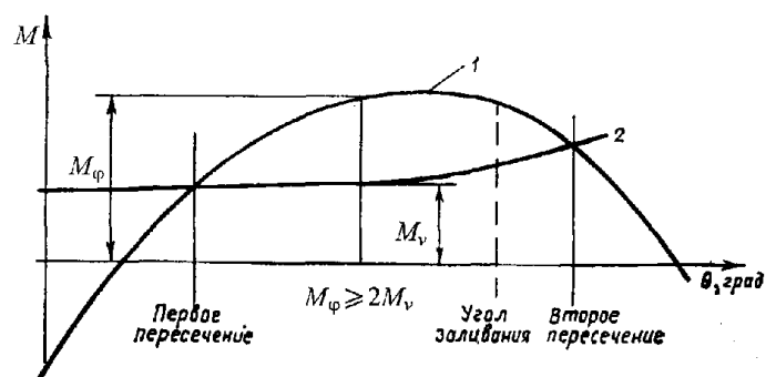
Рис. 2.5.5.4 Кривые восстанавливающего момента (1) и ветрового кренящего (2)
