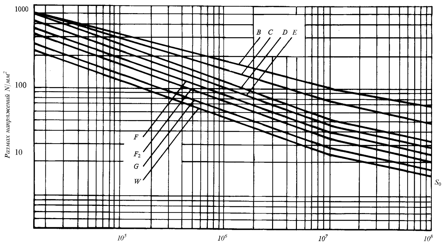
Рис. 2.4.4.8-1 Кривые усталости
