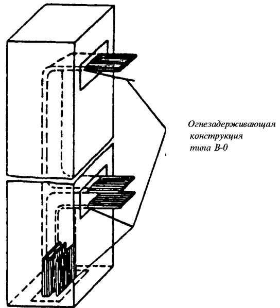
Рис. 16.8.4.3.1 Защита кабельной трассы полностью закрытой конструкцией В-0
