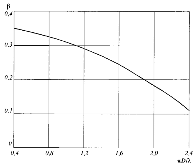
Рис. 3.3.2.1.8.2 Зависимость коэффициента \beta от \pi D/\lambda
