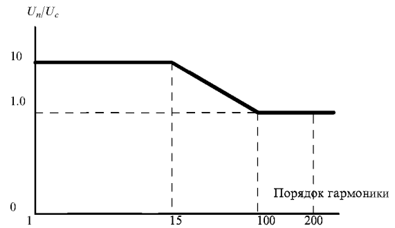
Рис. 2.2.1.2.2 График высших гармоник сети
