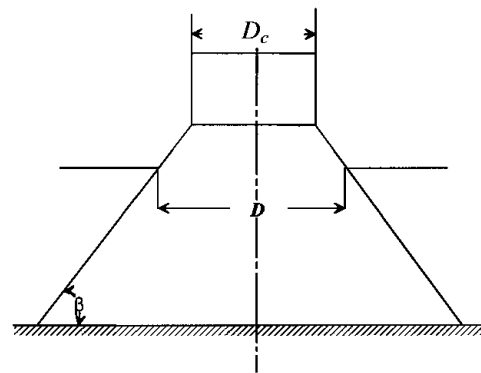
Рис. 3.3.2.3.5-3 Коническая преграда
