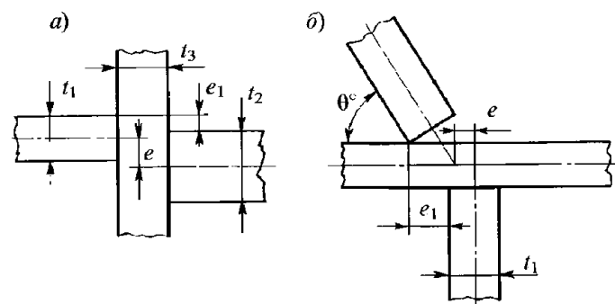
Рис. 2.7.1.11-2 Нарушение соосности деталей для крестообразных соединений:
