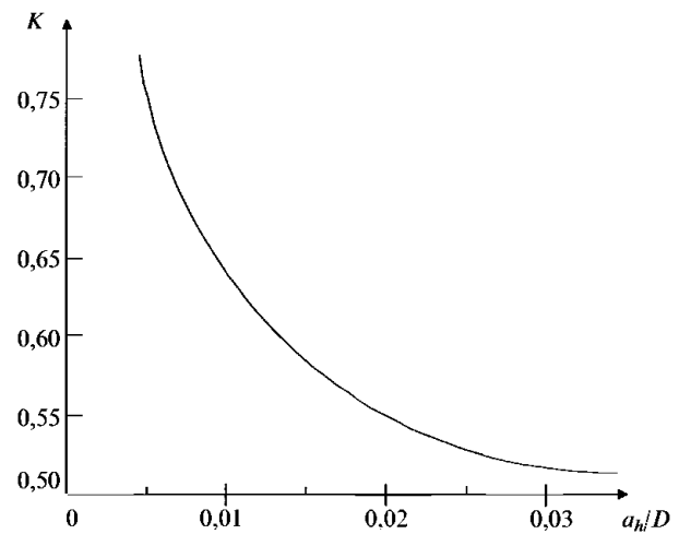
Рис. 3.3.2.3.5-2 Зависимость параметра формы K от отношения a_n/D
