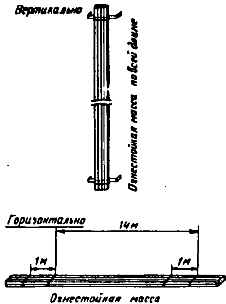
Рис. 16.8.4.3.2-1 Защита кабельной трассы огнестойкой массой
