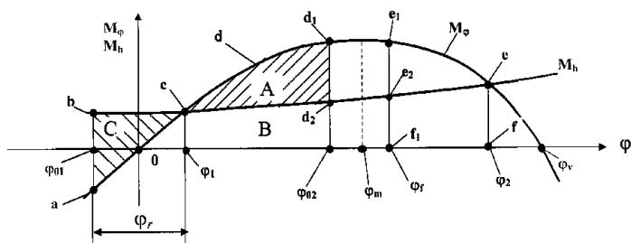
Рис. 3.1.1-1 Диаграмма статической устойчивости с учетом качки:
