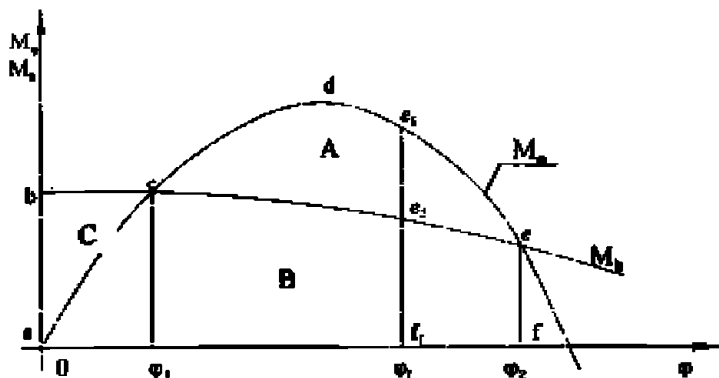
Рис. 3.1.1-2 Диаграмма статической устойчивости без учета качки
