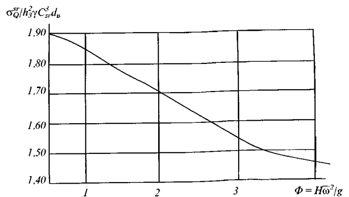
Рис. 3.1.4.13-1 Зависимость \sigma_Q^{sr}/h_3^2 \gamma C_{sr}^3 d_b от параметра
