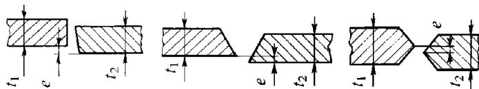
Рис. 2.7.1.11-1 Нарушение соосности деталей для стыковых соединений:
