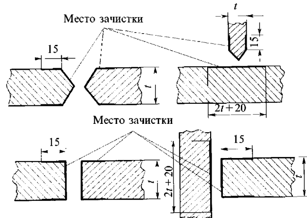
Рис. 2.8.10 Схема зачистки кромок стыкуемых деталей
