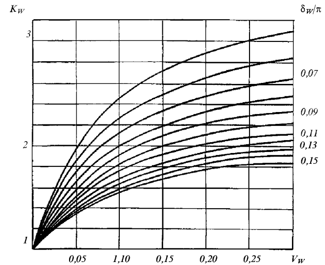
Рис. 3.1.3.2 Коэффициент динамичности ветровых нагрузок
