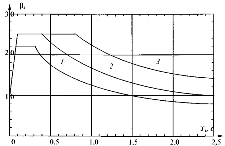
Рис. 3.3.2.4.11 Коэффициенты динамичности \beta(T_i) : кривая 1 — для грунтов I категории; кривая 2 — для грунтов I — II, II, II — III, III категорий при толщине верхнего слоя грунта не более 20 м; кривая 3 — для грунтов I — II, II, II — III, III категорий при толщине верхнего слоя грунта не менее 40 м
