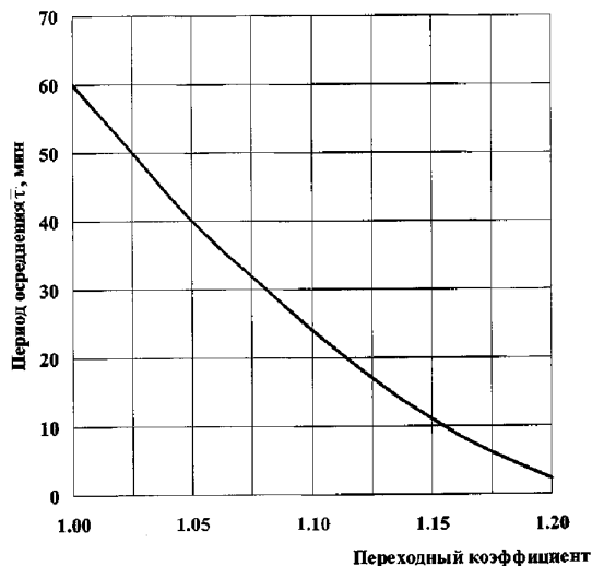
Рис. 2.2.2.4 График переходных коэффициентов v_t/v_{60}
