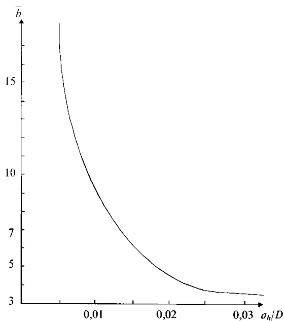
Рис. 3.3.2.3.5-1 Зависимость параметра \bar{b} от отношения a_n/D
