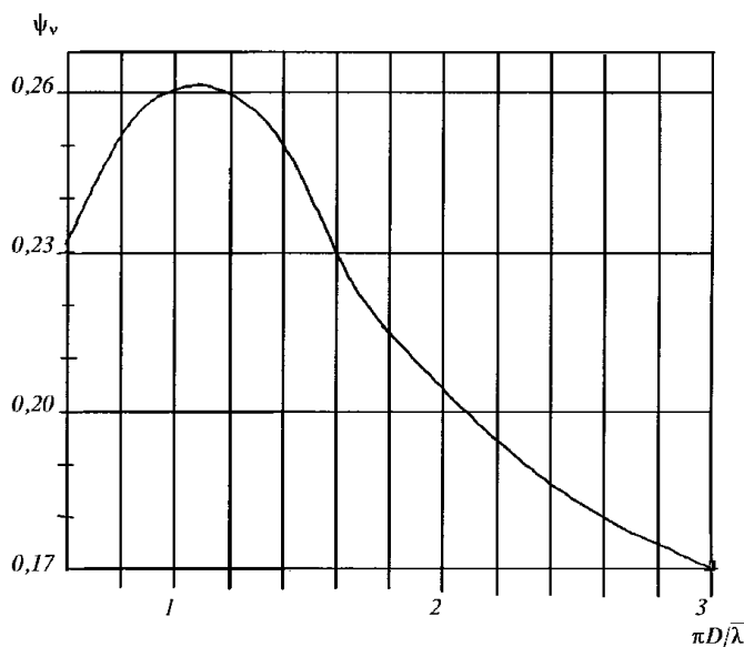
Рис. 3.3.2.1.7 Значение параметра \psi_v дополнительного опрокидывающего момента
