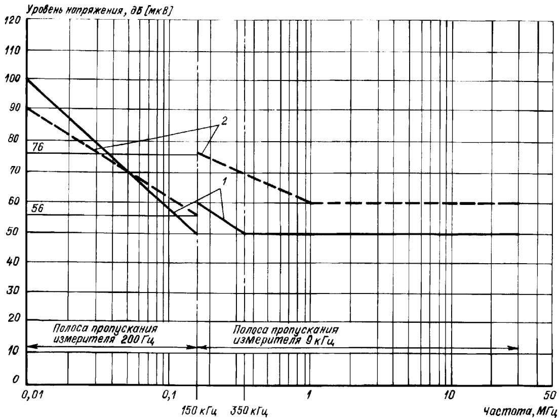
Рис. 2.2.1.4 Допустимые уровни напряжения помех:
