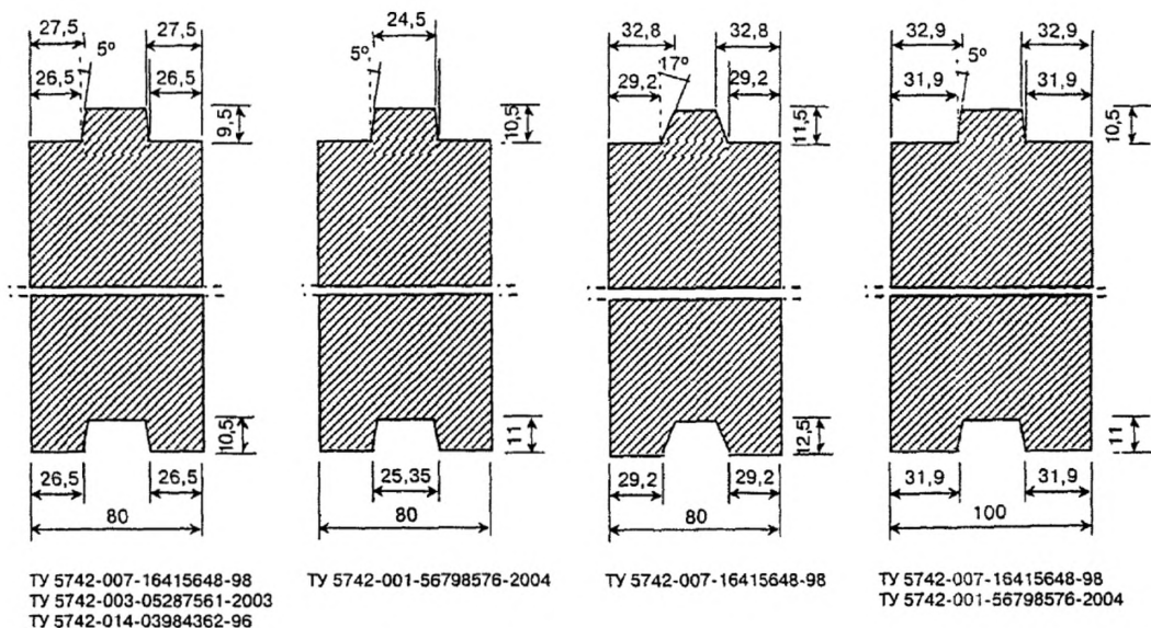
Рисунок 2. Типы пазогребневых плит
