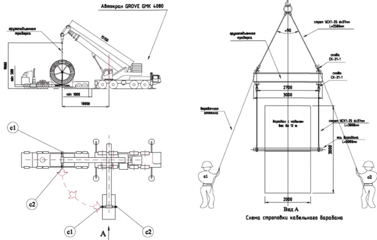
Рис. 2 Разгрузка и строповка барабана с кабелем
