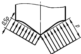
Рис. 2.7.8. Распределение давления в поперечном сечении экраноплана
