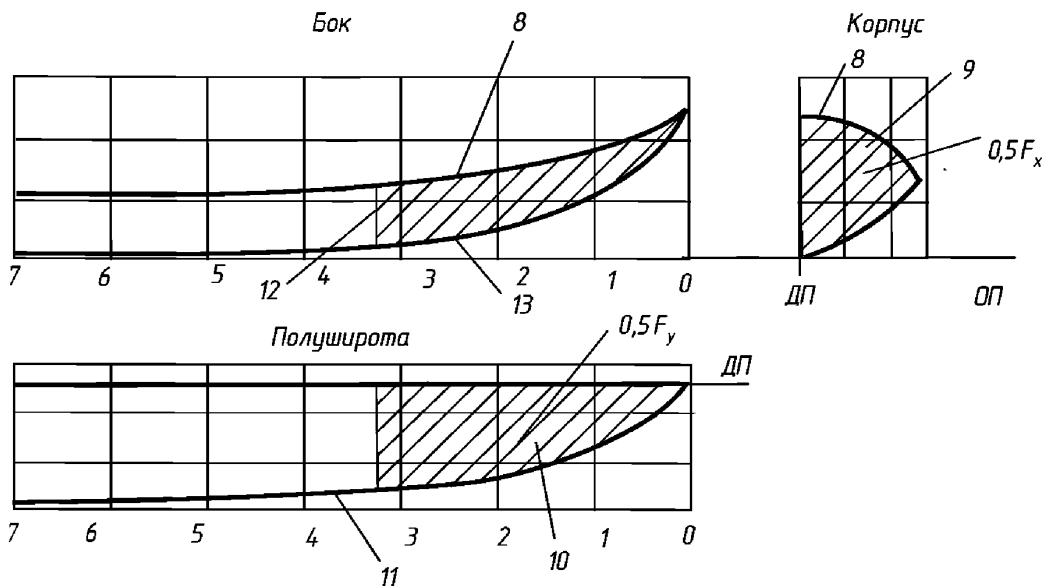
Рис. 2.3.8.2. Схема удара в носовую оконечность:
