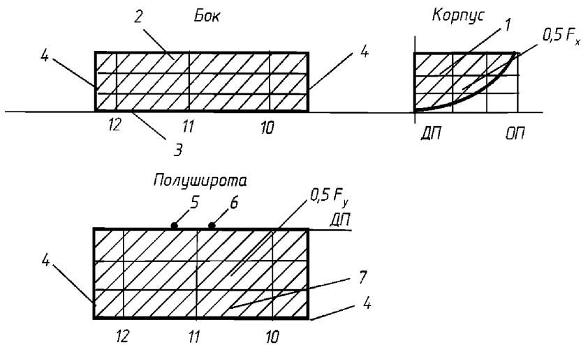
Рис. 2.3.9.2. Схема удара в район центра масс:
