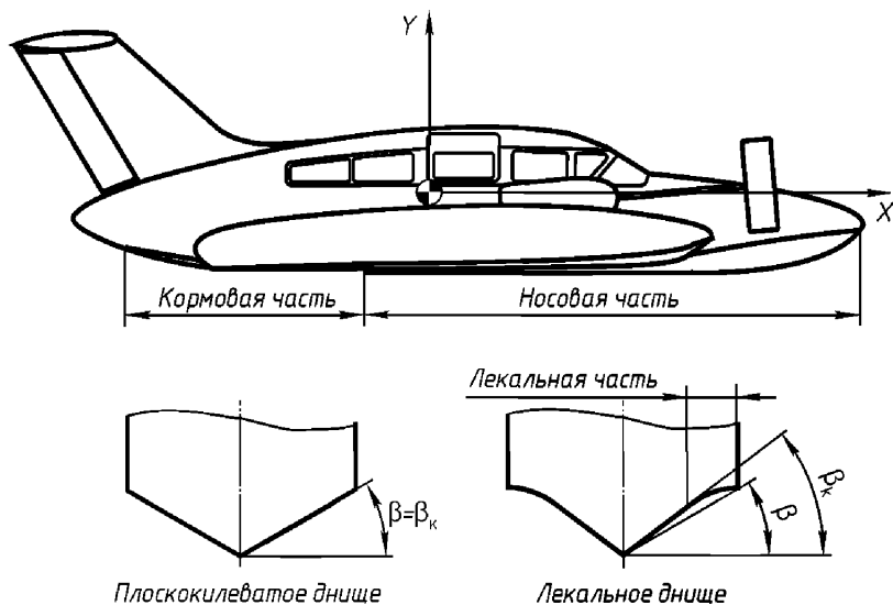
Рис. 2.7.4.1. Оси координат, углы килеватости, основные размеры экраноплана
