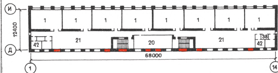
ПЛАН 3 ЭТАЖА
