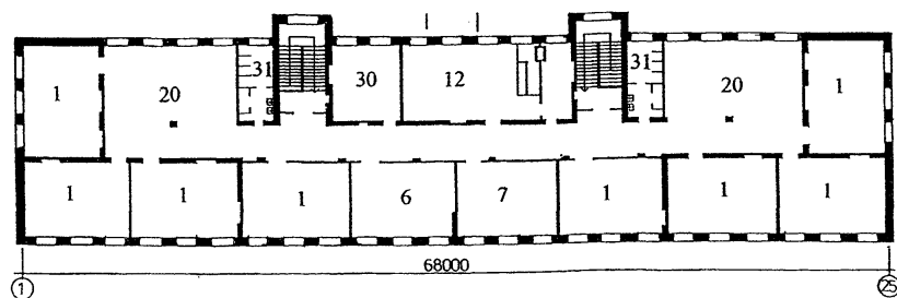
ПЛАН 3 ЭТАЖА
