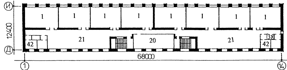
ПЛАН 3 ЭТАЖА
