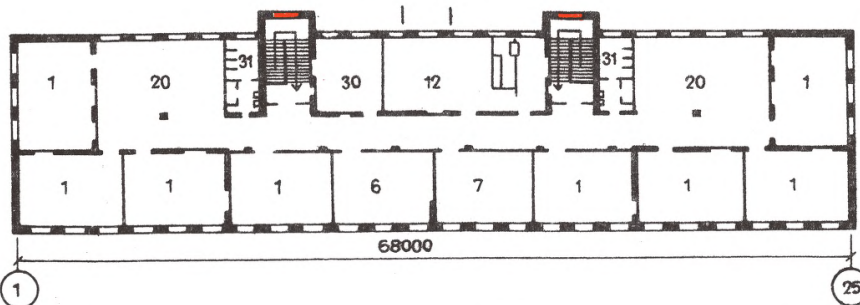
ПЛАН 3 ЭТАЖА
