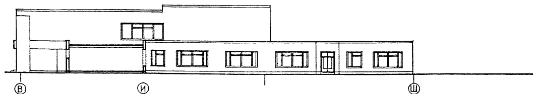
ФАСАД В-Ш
