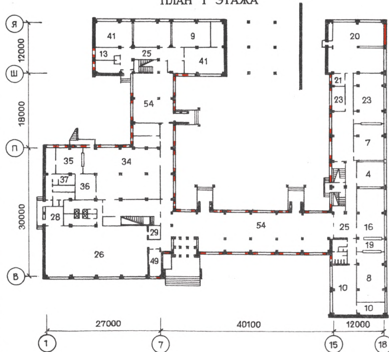
ПЛАН 1 ЭТАЖА
