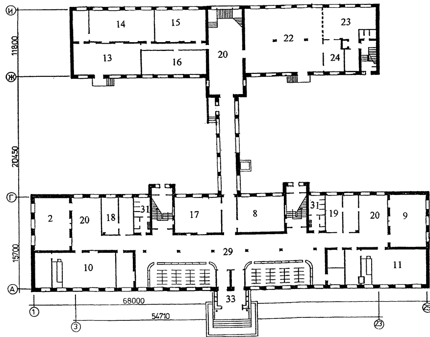
ПЛАН 3 ЭТАЖА
