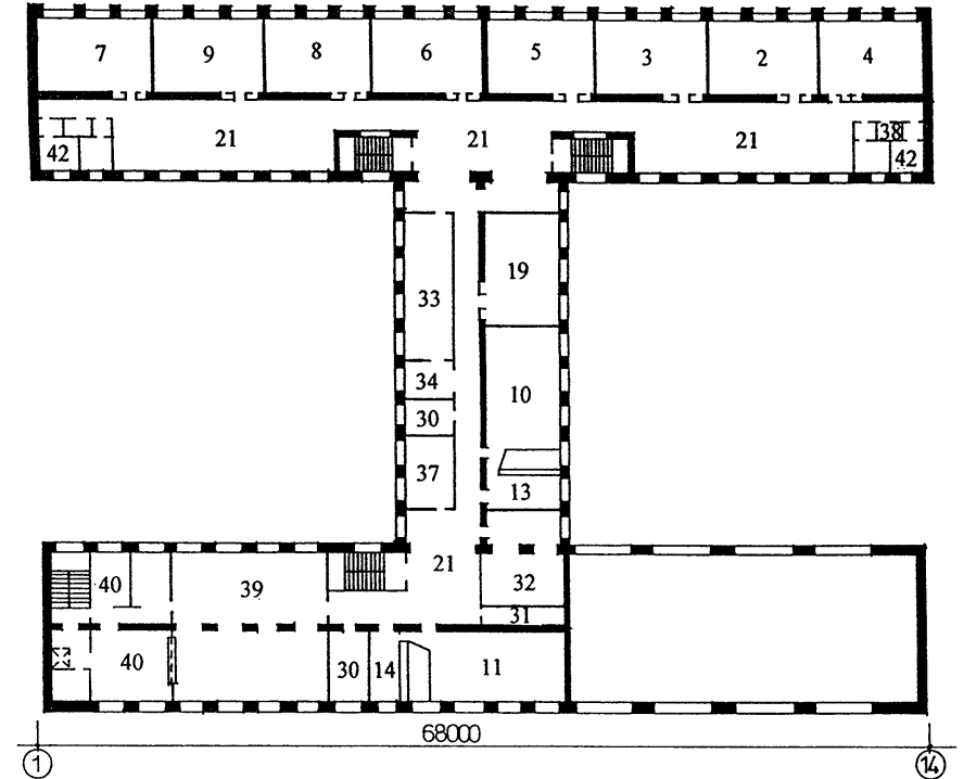
ПЛАН 2 ЭТАЖА
