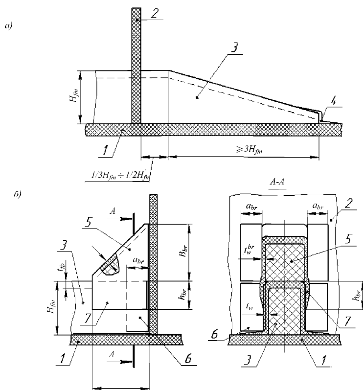
Рис. 3.19 Узлы окончания продольных балок П-образного профиля: а — на «ус» за переборкой (оформление прохода балки набора через переборку — см. рис. 3.18); б — на переборке с установкой кницы П-образного профиля; 1 — обшивка (настил); 2 — переборка; 3 — балка; 4 — заформовка конца балки набора; 5 — кница; 6 — накладка-угольник соединения стенки балки с переборкой; 7 — продолжение обформовки кницы на стенки балки набора; B_{br} \cong H_{fm} , t_{fp}^{br} \geq 0,8t_{fp} , t_w^{br} \cong t_w , t_{angl} \cong t_w , a_{br} \geq 12t_w , 1/2H_{fm} > h_{br} \geq 10t_w^{br}
