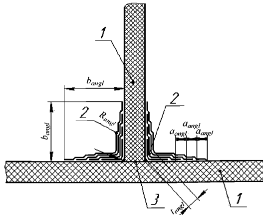
Рис. 3.34 Конструктивная схема углового формованного соединения: 1 — соединяемые связи; 2 — приформовочные угольники; 3 — поверхность контакта
