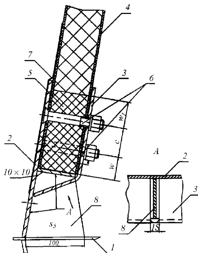
Рис. 3.52 Узел клеebolтового соединения панелей бортовых стенок надстройки с металлическим корпусом: 1 — палуба корпуса; 2 — комингс; 3 — накладная планка; 4 — панель бортовой стенки; 5 — пенопласт повышенной плотности; 6 — болты; 7 — обформовка; 8 — кница
