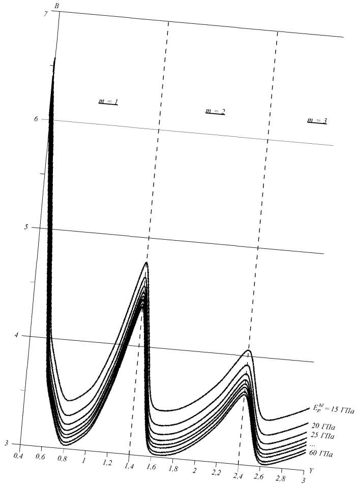
Рис. 4 Значения коэффициента B при G_{12}^N = 5 \text{ ГПа}
