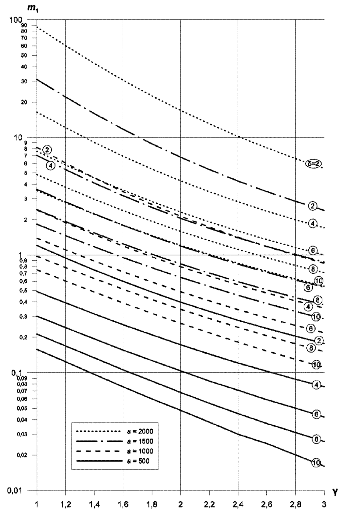
Рис. 12 Значения коэффициента m_1 при \eta = 800
