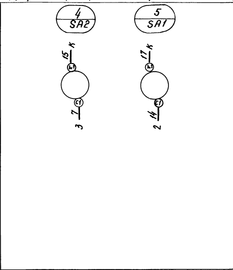
Дверь шкафа (Вид со стороны монтажа)
