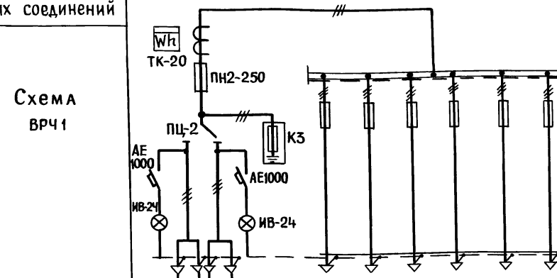
Схема межпанельных соединений
