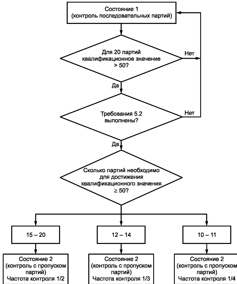
Рисунок 2 — Блок-схема определения начальной частоты контроля
