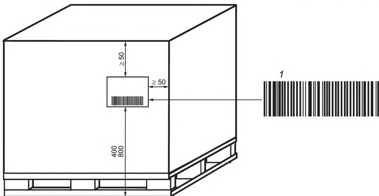
Рисунок 1 — Размещение этикетки на поддоне
